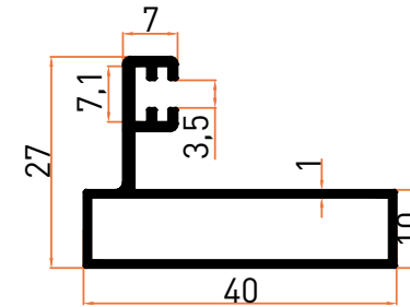
Profil No | 2246 Ağırlık / Weight: 0,387 kg/m
