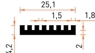
Profil No | 5016 Ağırlık / Weight: 0,223 kg/m
