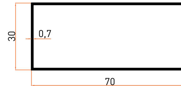
Profil No | 6460 Ağırlık / Weight: 0,374 kg/m
