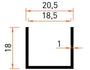
Profil No | 6796 Ağırlık / Weight: 0,148 kg/m
