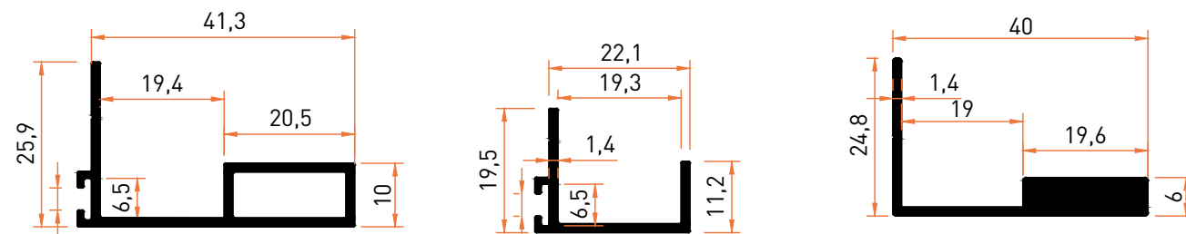
Profil No | 2214 Ağırlık / Weight: 0,403 kg/m Profil No | 2202 Ağırlık / Weight: 0,211 kg/m Profil No | 2222 Ağırlık / Weight: 0,484 kg/m
