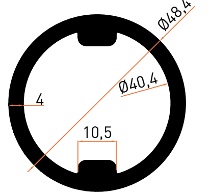
Profil No | 1639 Ağırlık / Weight: 1,744 kg/m
