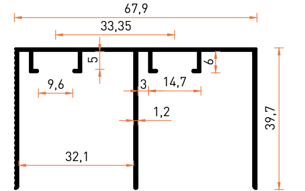
Profil No | 5550 Ağırlık / Weight: 0,631 kg/m
