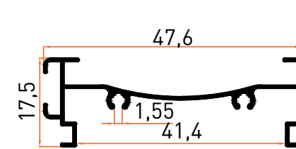
Profil No | 5612 Ağırlık / Weight: 0,217 kg/m
