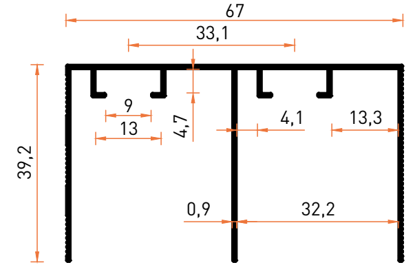
Profil No | 7520 Ağırlık / Weight: 0,500 kg/m
