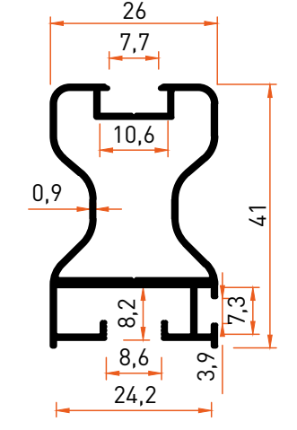
Profil No | 7004 Ağırlık / Weight: 0,456 kg/m
