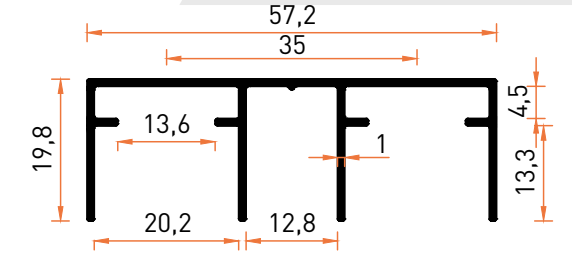
Profil No | 6794 Ağırlık / Weight: 0,395 kg/m
