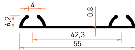
Profil No | 5513 Ağırlık / Weight: 0,202 kg/m
