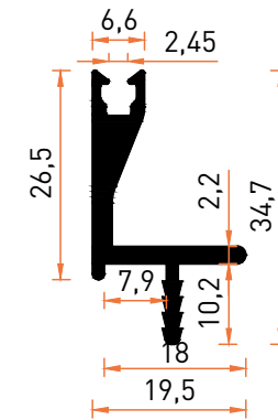
Profil No | 7118 Ağırlık / Weight: 0,384 kg/m
