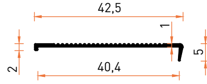
Profil No | 6734 Ağırlık / Weight: 0,108 kg/m
