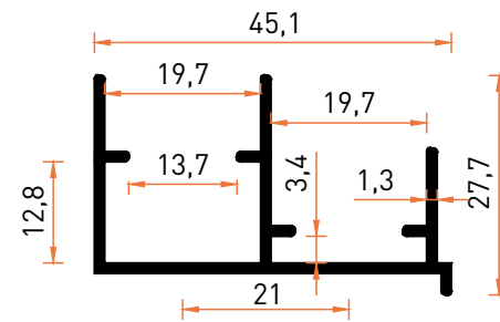
Profil No | 2591 Ağırlık / Weight: 0,441 kg/m
