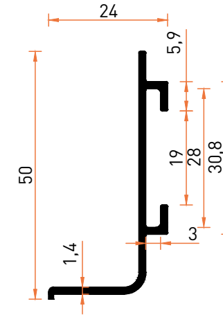
Profil No | 6165 Ağırlık / Weight: 0,320 kg/m
