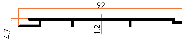
Profil No | 1015 Ağırlık / Weight: 0,357 kg/m
