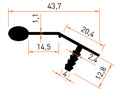
Profil No | 6897 Ağırlık / Weight: 0,360 kg/m
