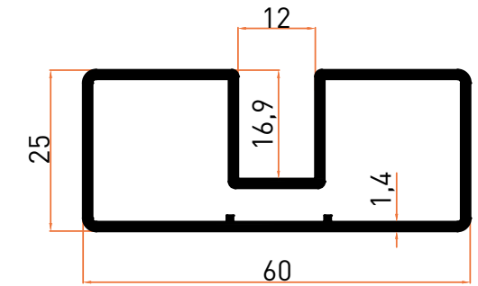
Profil No | 5943 Ağırlık / Weight: 0,746 kg/m
