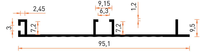
Profil No | 6611 Ağırlık / Weight: 0,417 kg/m
