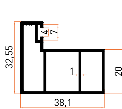
Profil No | 5895 Ağırlık / Weight: 0,524 kg/m
