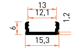
Profil No | 6931 Ağırlık / Weight: 0,081 kg/m
