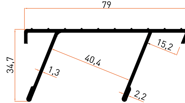
Profil No | 5113 Ağırlık / Weight: 0,631 kg/m
