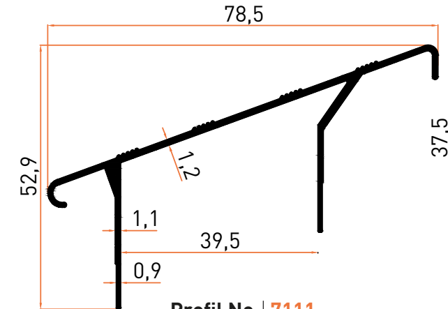
Profil No | 7111 Ağırlık / Weight: 0,512 kg/m
