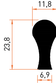
Profil No | 5366 Ağırlık / Weight: 0,488 kg/m
