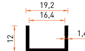
Profil No | 2850 Ağırlık / Weight: 0,153 kg/m
