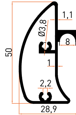
Profil No | 5783 Ağırlık / Weight: 0,507 kg/m
