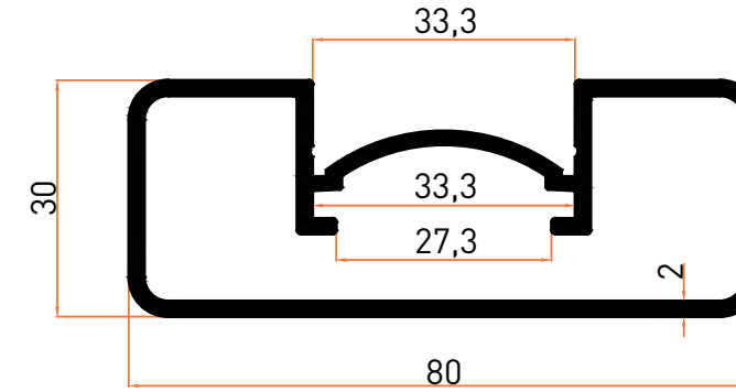
Profil No | 2922 Ağırlık / Weight: 1,335 kg/m
