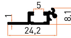
Profil No | 5801 Ağırlık / Weight: 0,125 kg/m
