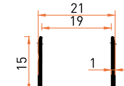
Profil No | 2744 Ağırlık / Weight: 0,129 kg/m
