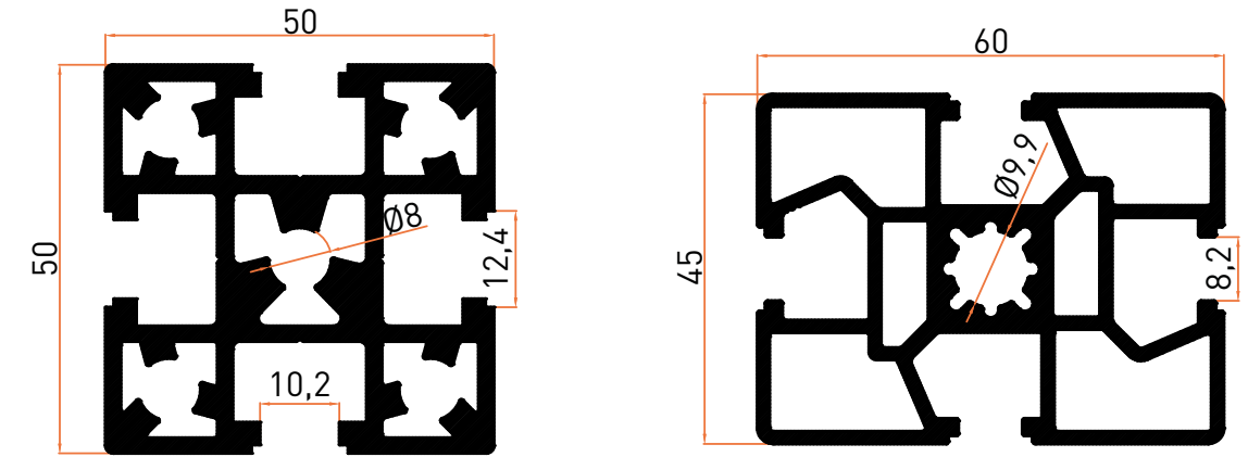
Profil No | 6902 Ağırlık / Weight: 2,597 kg/m
