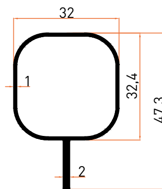
Profil No | 6474 Ağırlık / Weight: 0,374 kg/m
