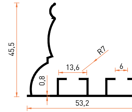
Profil No | 2563 Ağırlık / Weight: 0,344 kg/m
