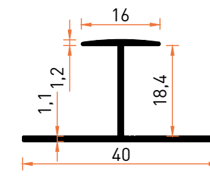
Profil No | 7417 Ağırlık / Weight: 0,217 kg/m
