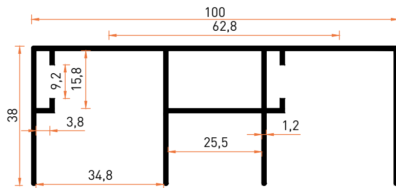
Profil No | 5022 Ağırlık / Weight: 0,960 kg/m
