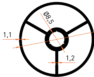
Profil No | 7343 Ağırlık / Weight: 0,663 kg/m
