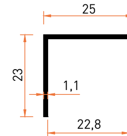
Profil No | 6425 Ağırlık / Weight: 0,203 kg/m
