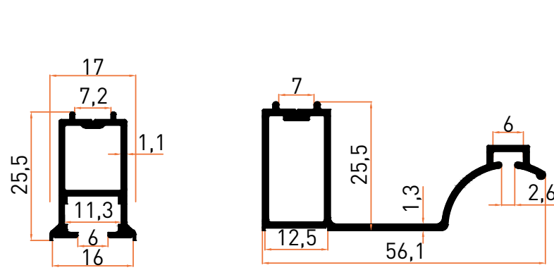
Profil No | 12228 Ağırlık / Weight: 0,260 kg/m
