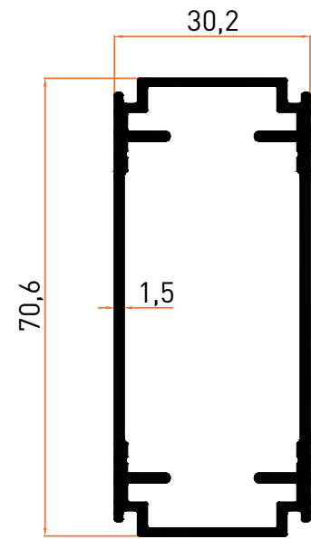
Profil No | 2587 Ağırlık / Weight: 0,933 kg/m
