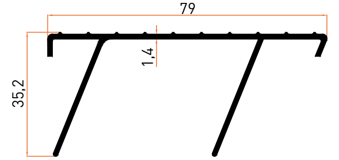
Profil No | 6731 Ağırlık / Weight: 0,597 kg/m
