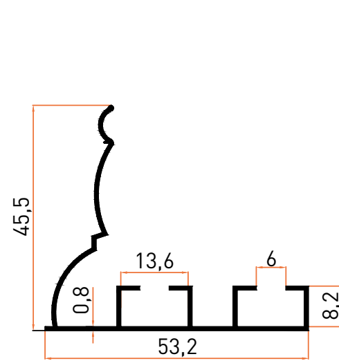
Profil No | 2563 Ağırlık / Weight: 0,344 kg/m
