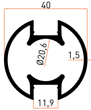
Profil No | 1607 Ağırlık / Weight: 0,724 kg/m
