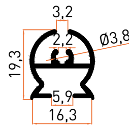
Profil No | 12295 Ağırlık / Weight: 0,238 kg/m
