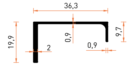
Profil No | 7676 Ağırlık / Weight: 0,218 kg/m
