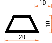
Profil No | 5390 Ağırlık / Weight: 0,153 kg/m
