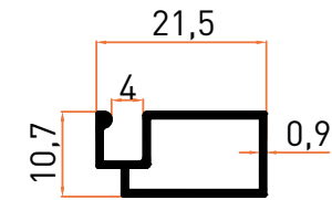
Profil No | 2503 Ağırlık / Weight: 0,152 kg/m
