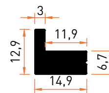
Profil No | 1580 Ağırlık / Weight: 0,331 kg/m
