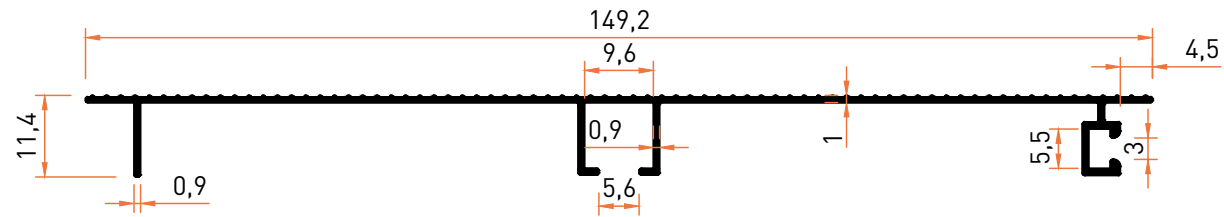
Profil No | 7167 Ağırlık / Weight: 0,481 kg/m
