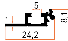
Profil No | 5519 Ağırlık / Weight: 0,125 kg/m
