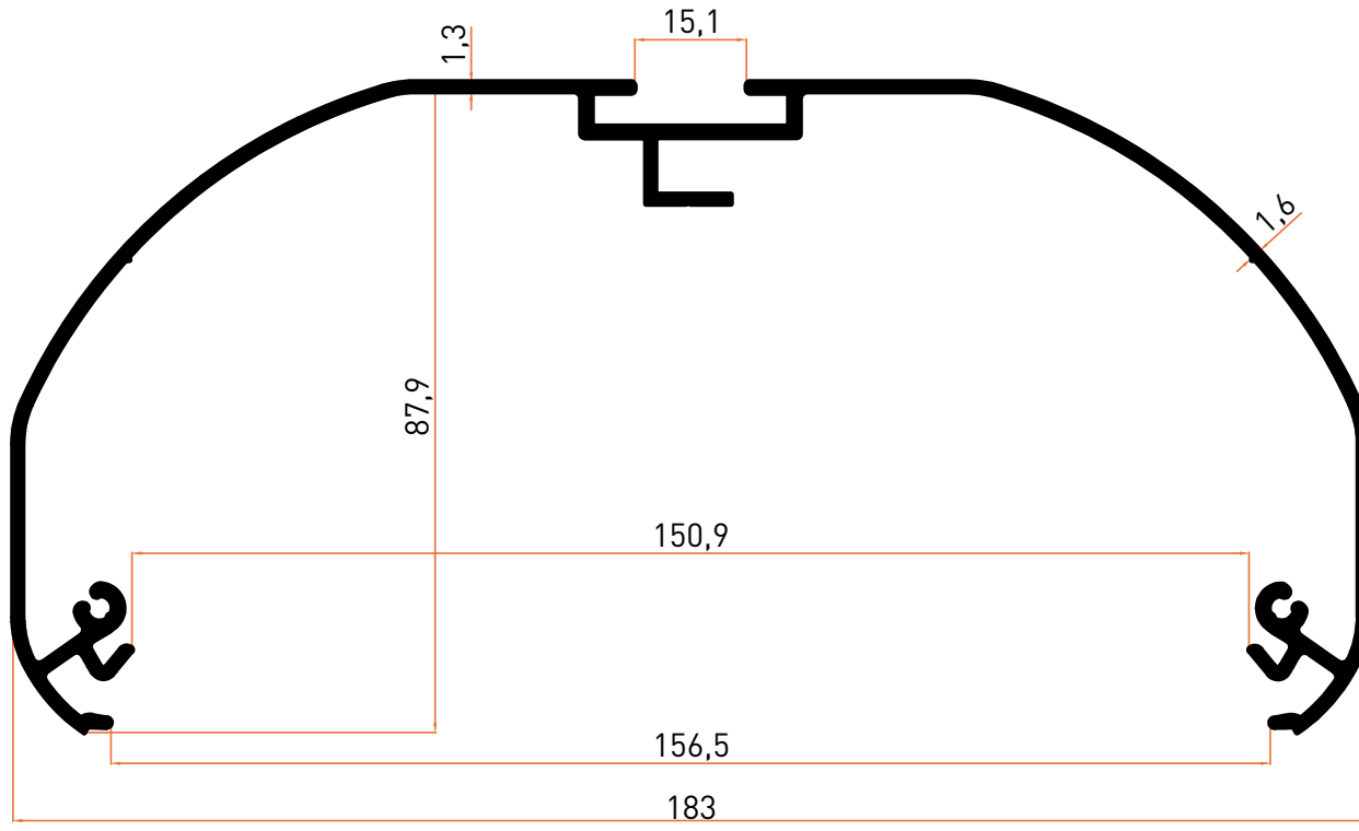
Profil No | 4001 Ağırlık / Weight: 1,553 kg/m
