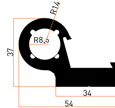
Profil No | 2579 Ağırlık / Weight: 2,013 kg/m
