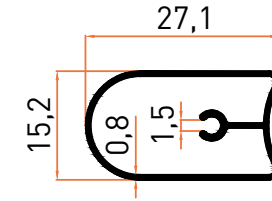
Profil No | 5608 Ağırlık / Weight: 0,192 kg/m
