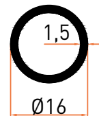
Profil No | 1605 Ağırlık / Weight: 0,185 kg/m
