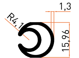
Profil No | 5377 Ağırlık / Weight: 0,228 kg/m
