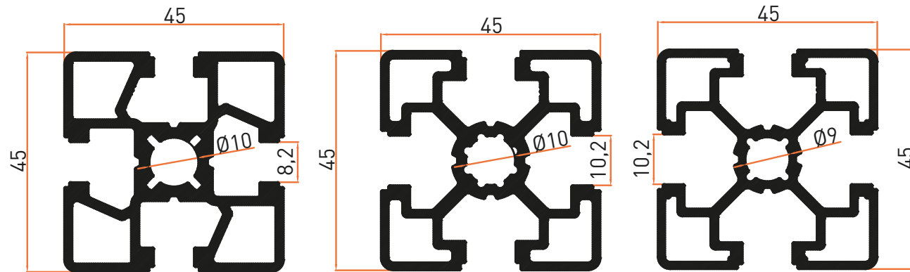
Profil No | 6986 Ağırlık / Weight: 1,707 kg/m
