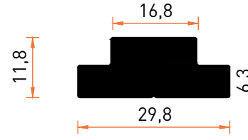
Profil No | 5506 Ağırlık / Weight: 0,759 kg/m
