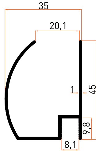
Profil No | 5782 Ağırlık / Weight: 0,367 kg/m
