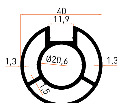
Profil No | 1625 Ağırlık / Weight: 0,818 kg/m
