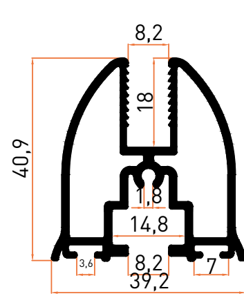
Profil No | 5357 Ağırlık / Weight: 0,914 kg/m
