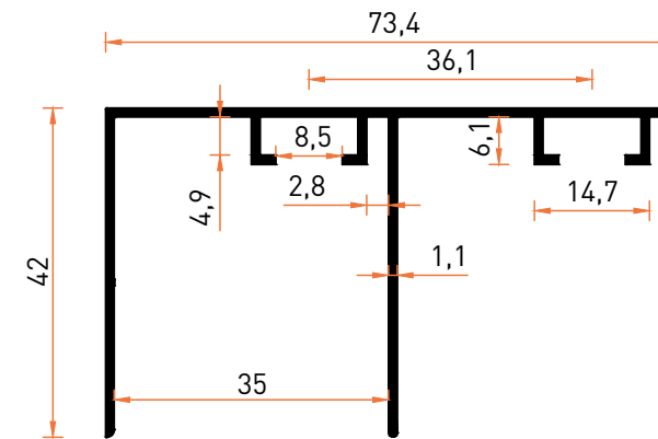
Profil No | 5940 Ağırlık / Weight: 0,678 kg/m
