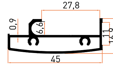
Profil No | 6817 Ağırlık / Weight: 0,361 kg/m
