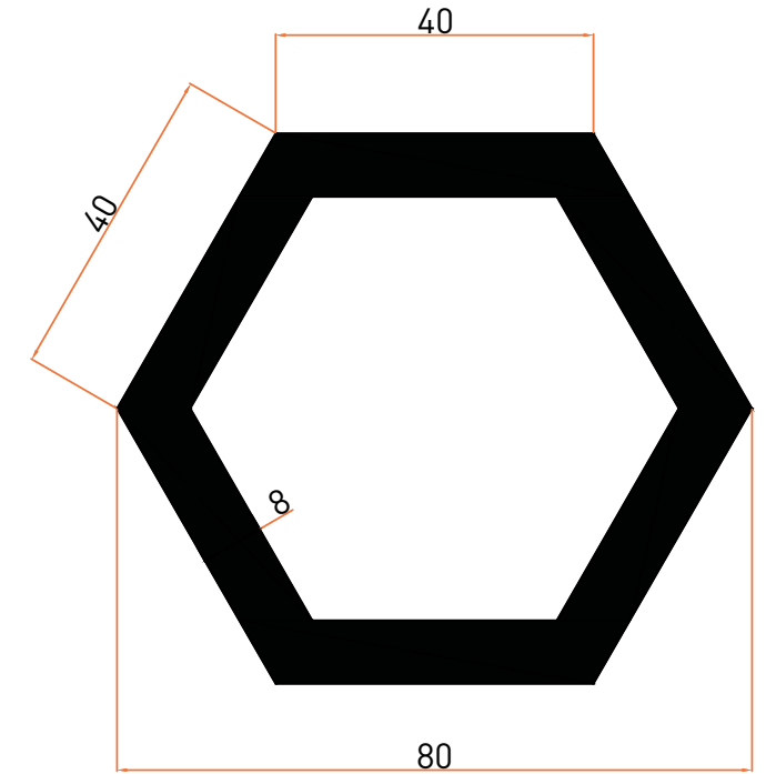
Profil No | 2670 Ağırlık / Weight: 4,602 kg/m
