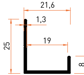
Profil No | 2207 Ağırlık / Weight: 0,182 kg/m
