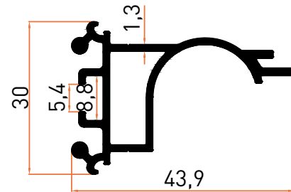
Profil No | 5941 Ağırlık / Weight: 0,500 kg/m
