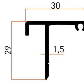
Profil No | 2625 Ağırlık / Weight: 0,277 kg/m
