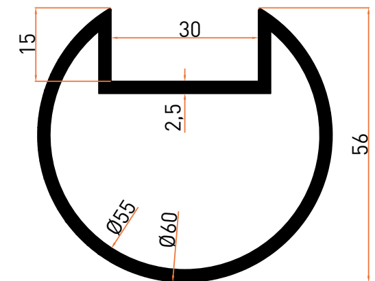
Profil No | 5260 Ağırlık / Weight: 1,398 kg/m
