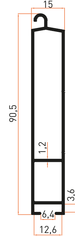
Profil No | 2757 Ağırlık / Weight: 0,719 kg/m
