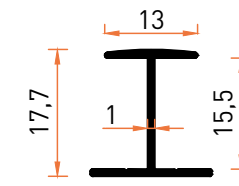
Profil No | 7383 Ağırlık / Weight: 0,132 kg/m
