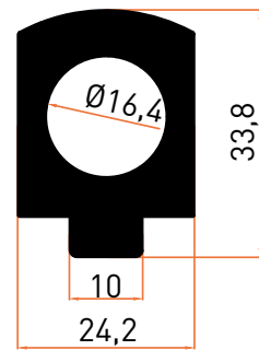
Profil No | 1611 Ağırlık / Weight: 1,365 kg/m
