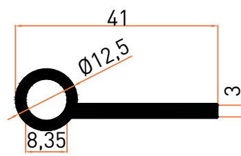
Profil No | 4014 Ağırlık / Weight: 0,434 kg/m
