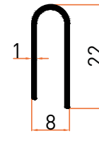
Profil No | 2559 Ağırlık / Weight: 0,122 kg/m
