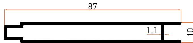
Profil No | 1014 Ağırlık / Weight: 0,564 kg/m
