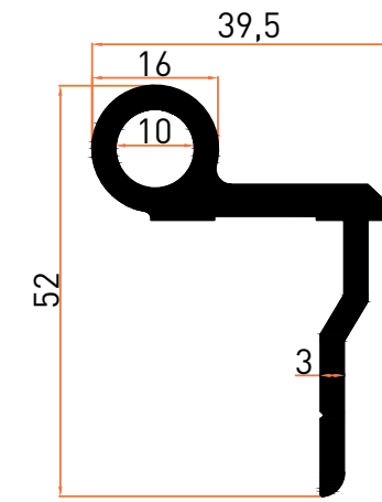
Profil No | 2578 Ağırlık / Weight: 0,952 kg/m
