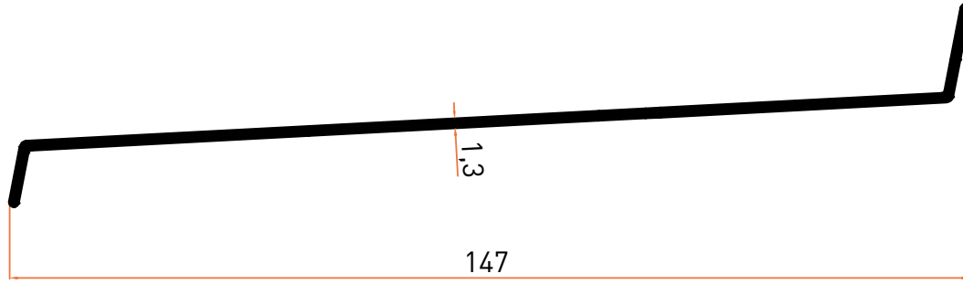
Profil No | 3153 Ağırlık / Weight: 0,582 kg/m
