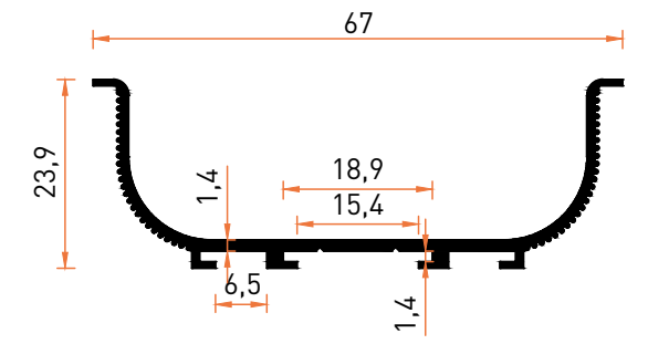
Profil No | 7079 Ağırlık / Weight: 0,400 kg/m
