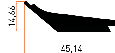
Profil No | 2582 Ağırlık / Weight: 0,740 kg/m
