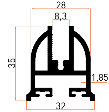
Profil No | 2245 Ağırlık / Weight: 0,905 kg/m
