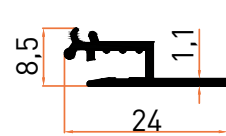
Profil No | 5517 Ağırlık / Weight: 0,130 kg/m
