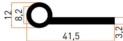
Profil No | 4047 Ağırlık / Weight: 0,427 kg/m
