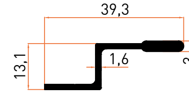
Profil No | 2508 Ağırlık / Weight: 0,256 kg/m
