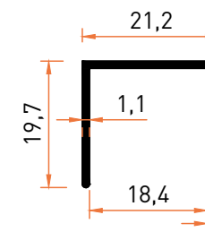
Profil No | 6737 Ağırlık / Weight: 0,194 kg/m
