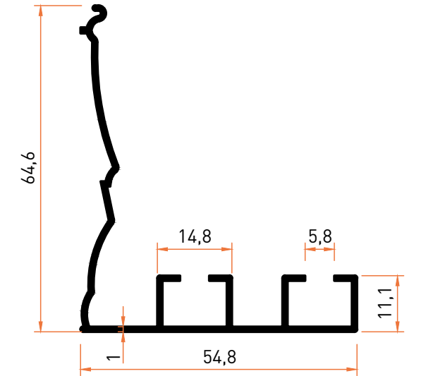
Profil No | 2545 Ağırlık / Weight: 0,503 kg/m
