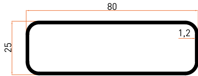
Profil No | 6729 Ağırlık / Weight: 0,637 kg/m
