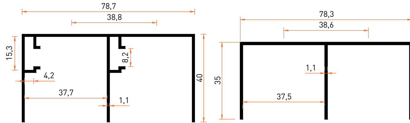
Profil No | 7304 Ağırlık / Weight: 0,678 kg/m
