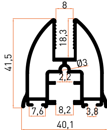
Profil No | 5059 Ağırlık / Weight: 0,842 kg/m
