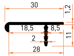
Profil No | 6662 Ağırlık / Weight: 0,154 kg/m
