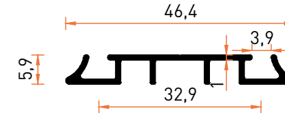
Profil No | 2231 Ağırlık / Weight: 0,223 kg/m
