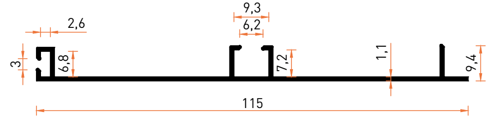
Profil No | 6797 Ağırlık / Weight: 0,471 kg/m
