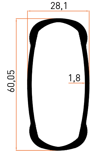
Profil No | 5249 Ağırlık / Weight: 0,879 kg/m
