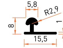
Profil No | 6885 Ağırlık / Weight: 0,100 kg/m
