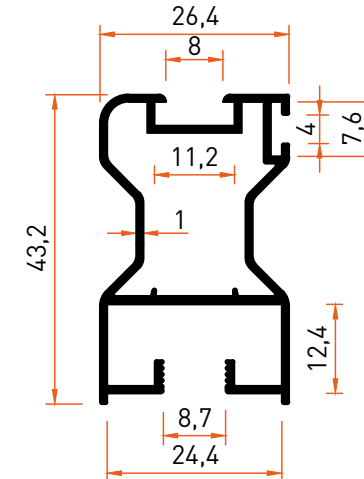
Profil No | 2220 Ağırlık / Weight: 0,510 kg/m
