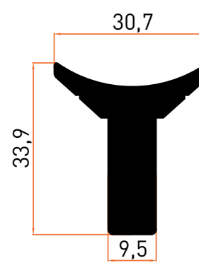
Profil No | 1628 Ağırlık / Weight: 1,028 kg/m
