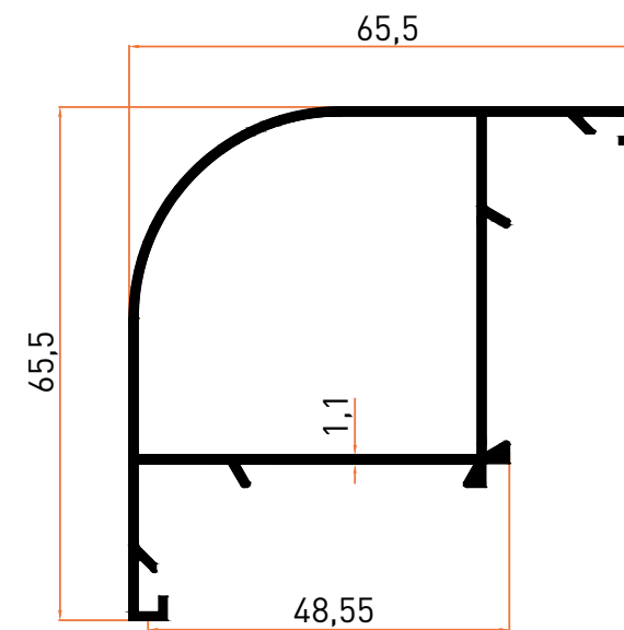
Profil No | 1011 Ağırlık / Weight: 0,719 kg/m
