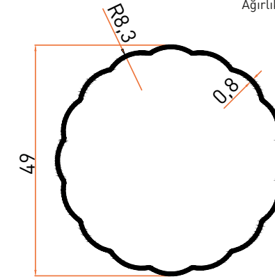
Profil No | 5171 Ağırlık / Weight: 0,332 kg/m
