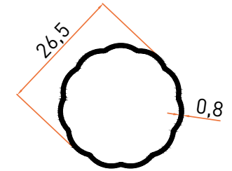
Profil No | 5172 Ağırlık / Weight: 0,175 kg/m
