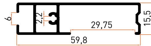
Profil No | 12240 Ağırlık / Weight: 0,411 kg/m
