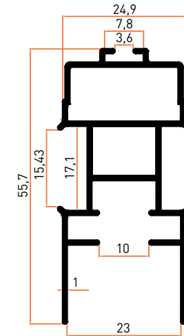
Profil No | 5722 Ağırlık / Weight: 0,515 kg/m
