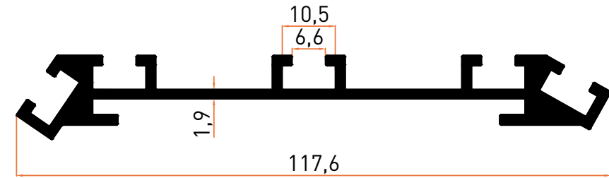
Profil No | 2669 Ağırlık / Weight: 1,312 kg/m
