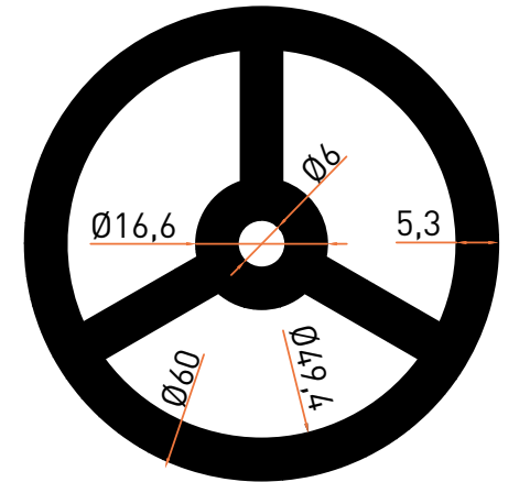
Profil No | 1638 Ağırlık / Weight: 3,689 kg/m
