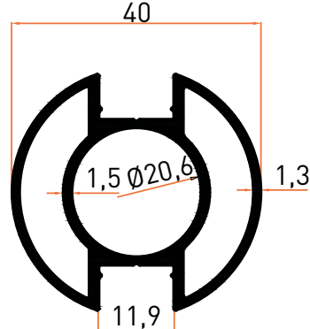
Profil No | 1626 Ağırlık / Weight: 0,796 kg/m
