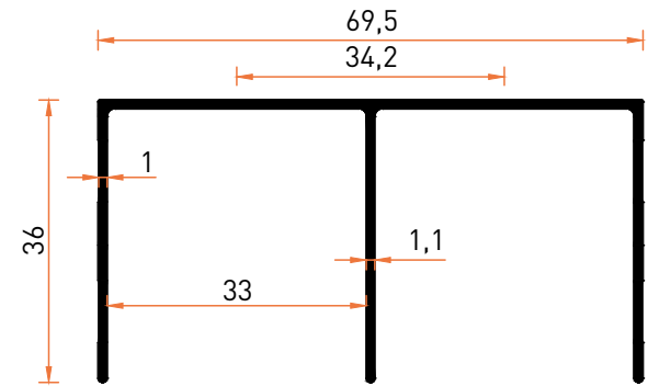
Profil No | 5204 Ağırlık / Weight: 0,521 kg/m
