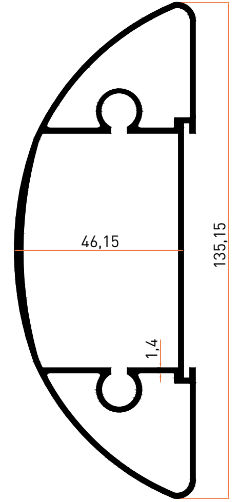
Profil No | 2540 Ağırlık / Weight: 1,805 kg/m
