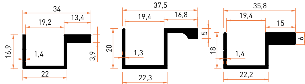
Profil No | 2224 Ağırlık / Weight: 0,327 kg/m Profil No | 2206 Ağırlık / Weight: 0,370 kg/m Profil No | 2208 Ağırlık / Weight: 0,435 kg/m
