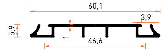
Profil No | 2232 Ağırlık / Weight: 0,268 kg/m
