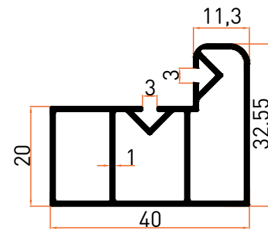
Profil No | 5894 Ağırlık / Weight: 0,873 kg/m
