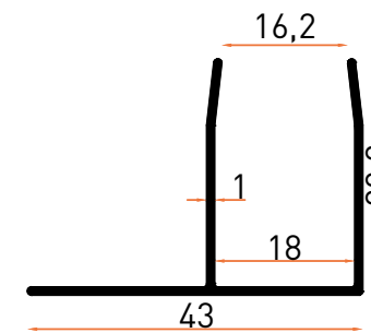
Profil No | 7117 Ağırlık / Weight: 0,272 kg/m
