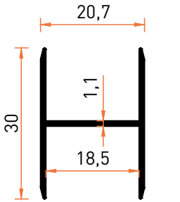
Profil No | 7431 Ağırlık / Weight: 0,227 kg/m
