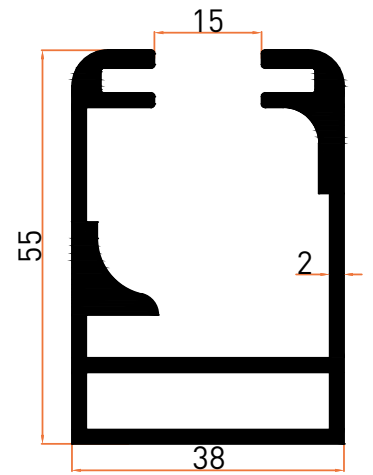
Profil No | 2244 Ağırlık / Weight: 1,417 kg/m
