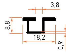
Profil No | 7318 Ağırlık / Weight: 0,126 kg/m
