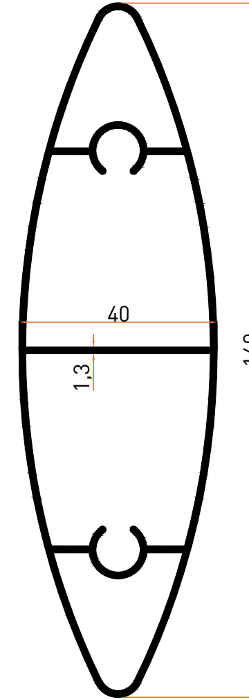
Profil No | 2548 Ağırlık / Weight: 1,510 kg/m
