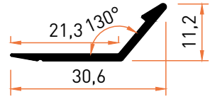
Profil No | 6881 Ağırlık / Weight: 0,123 kg/m
