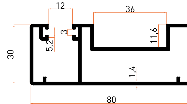
Profil No | 5942 Ağırlık / Weight: 1,034 kg/m
