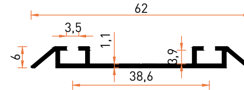
Profil No | 5208 Ağırlık / Weight: 0,269 kg/m
