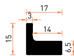
Profil No | 6257 Ağırlık / Weight: 0,371 kg/m
