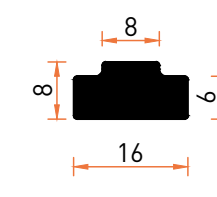
Profil No | 6249 Ağırlık / Weight: 0,304 kg/m
