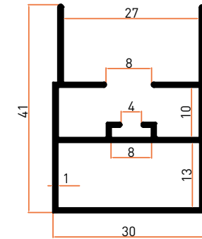
Profil No | 5723 Ağırlık / Weight: 0,421 kg/m
