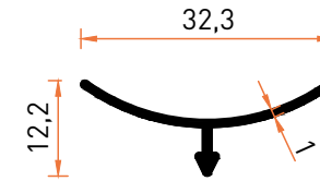
Profil No | 7382 Ağırlık / Weight: 0,119 kg/m
