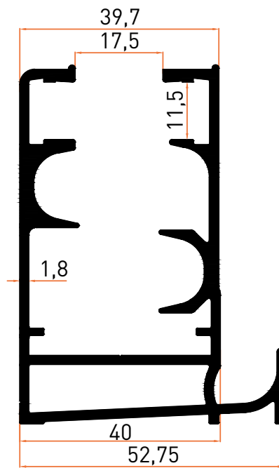
Profil No | 5889 Ağırlık / Weight: 1,662 kg/m
