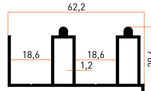
Profil No | 2780 Ağırlık / Weight: 0,704 kg/m
