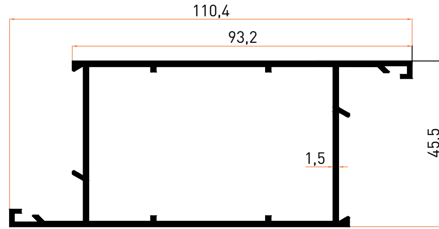
Profil No | 1008 Ağırlık / Weight: 1,203 kg/m
