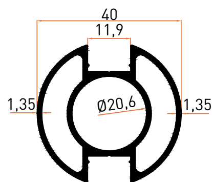
Profil No | 1622 Ağırlık / Weight: 0,786 kg/m
