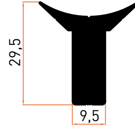
Profil No | 6167 Ağırlık / Weight: 0,792 kg/m
