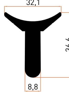
Profil No | 1616 Ağırlık / Weight: 0,973 kg/m
