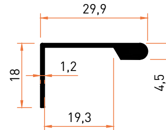
Profil No | 5006 Ağırlık / Weight: 0,217 kg/m
