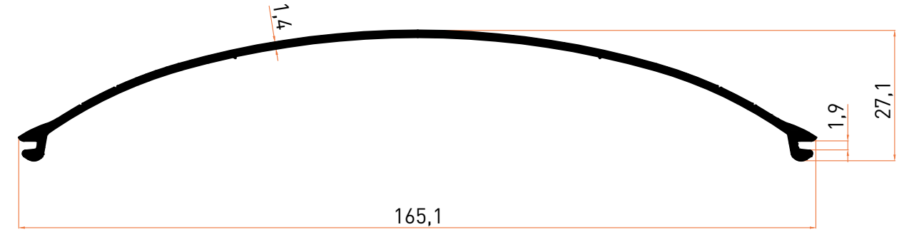
Profil No | 4002 Ağırlık / Weight: 0,732 kg/m
