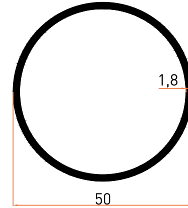
Profil No | 1627 Ağırlık / Weight: 0,739 kg/m
