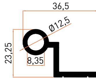
Profil No | 4005 Ağırlık / Weight: 0,459 kg/m
