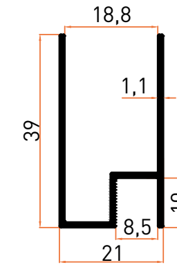
Profil No | 6276 Ağırlık / Weight: 0,314 kg/m
