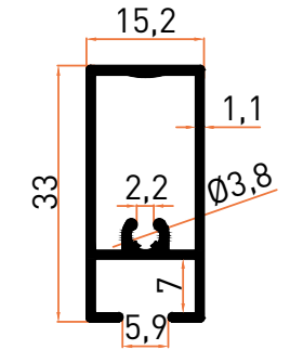
Profil No | 11767 Ağırlık / Weight: 0,333 kg/m
