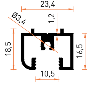
Profil No | 6753 Ağırlık / Weight: 0,310 kg/m
