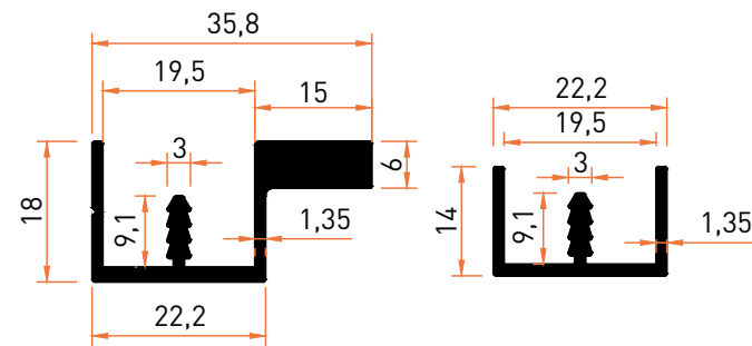
Profil No | 2210 Ağırlık / Weight: 0,511 kg/m Profil No | 2211 Ağırlık / Weight: 0,239 kg/m
