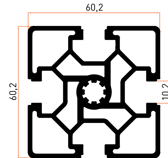
Profil No | 6980 Ağırlık / Weight: 2,634 kg/m
