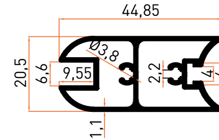
Profil No | 6121 Ağırlık / Weight: 0,596 kg/m
