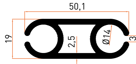
Profil No | 5134 Ağırlık / Weight: 0,969 kg/m
