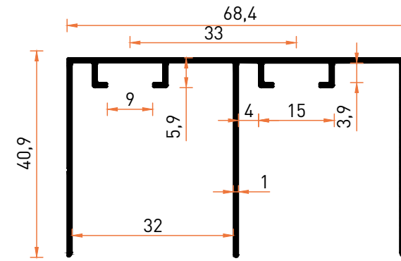
Profil No | 5546 Ağırlık / Weight: 0,596 kg/m
