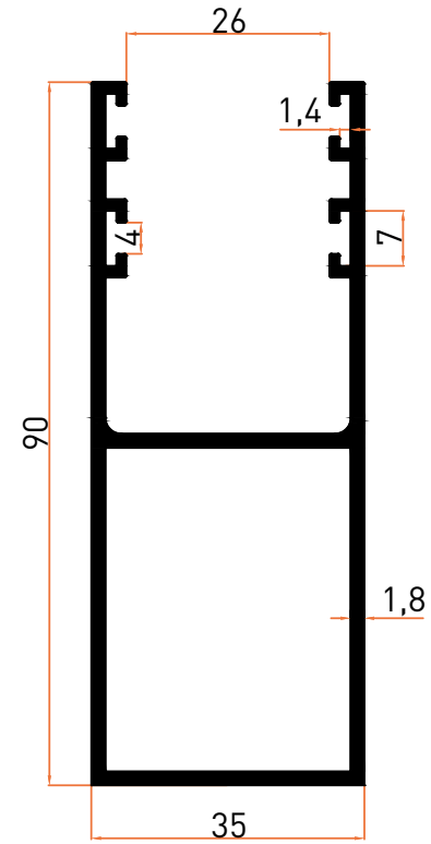
Profil No | 2756 Ağırlık / Weight: 1,318 kg/m
