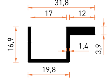
Profil No | 2596 Ağırlık / Weight: 0,330 kg/m
