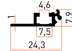
Profil No | 6726 Ağırlık / Weight: 0,126 kg/m
