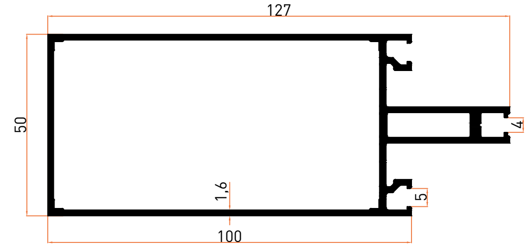
Profil No | 2960 Ağırlık / Weight: 1,764 kg/m
