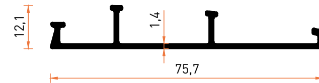
Profil No | 6047 Ağırlık / Weight: 0,442 kg/m
