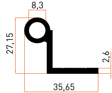
Profil No | 4022 Ağırlık / Weight: 0,487 kg/m
