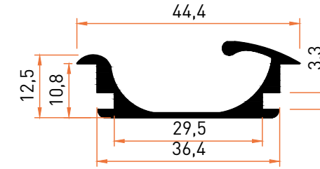
Profil No | 6862 Ağırlık / Weight: 0,375 kg/m
