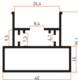
Profil No | 5775 Ağırlık / Weight: 0,486 kg/m
