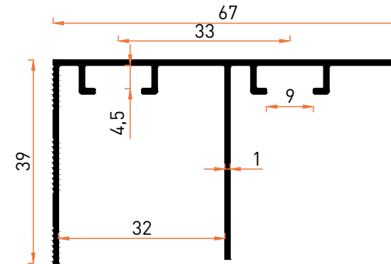
Profil No | 7041 Ağırlık / Weight: 0,558 kg/m
