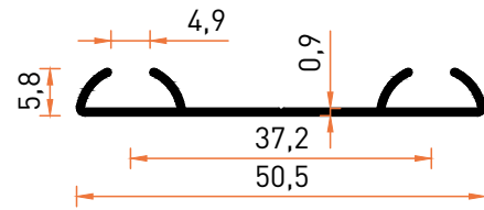
Profil No | 2564 Ağırlık / Weight: 0,188 kg/m
