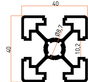
Profil No | 7133 Ağırlık / Weight: 1,059 kg/m
