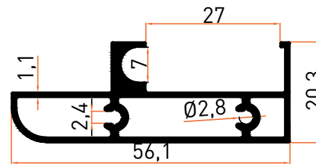
Profil No | 6275 Ağırlık / Weight: 0,615 kg/m
