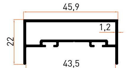
Profil No | 6938 Ağırlık / Weight: 0,468 kg/m
