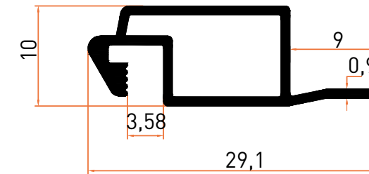
Profil No | 2511 Ağırlık / Weight: 0,358 kg/m
