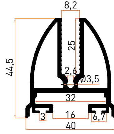
Profil No | 5890 Ağırlık / Weight: 0,958 kg/m
