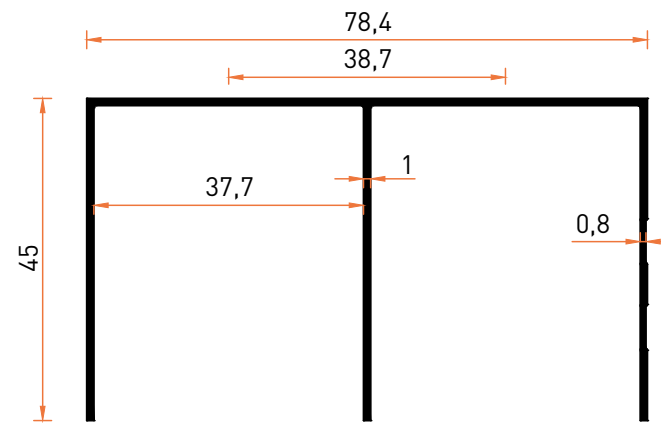
Profil No | 6776 Ağırlık / Weight: 0,563 kg/m
