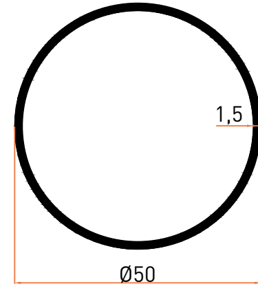
Profil No | 1601 Ağırlık / Weight: 0,619 kg/m
