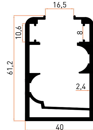
Profil No | 6229 Ağırlık / Weight: 1,413 kg/m
