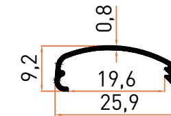
Profil No | 6715 Ağırlık / Weight: 0,087 kg/m
