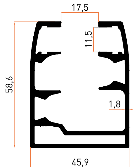
Profil No | 5892 Ağırlık / Weight: 1,493 kg/m
