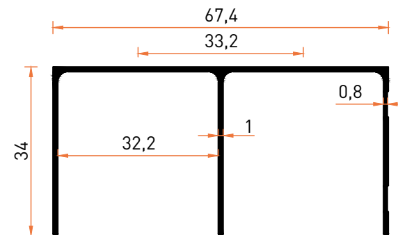
Profil No | 6612 Ağırlık / Weight: 0,453 kg/m
