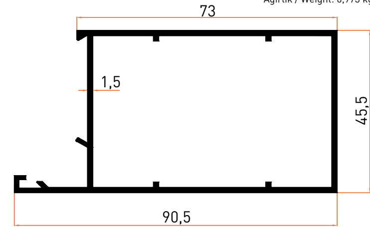
Profil No | 1018 Ağırlık / Weight: 1,072 kg/m
