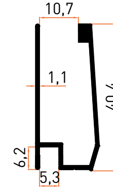
Profil No | 6919 Ağırlık / Weight: 0,326 kg/m
