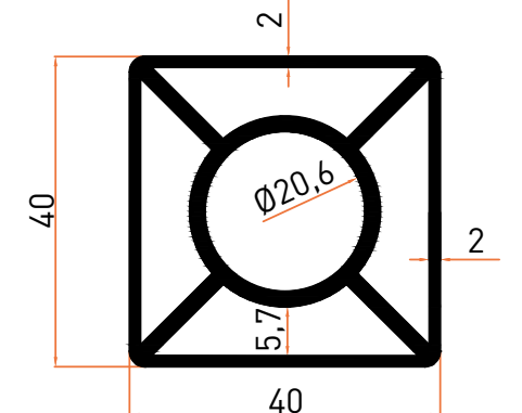
Profil No | 2784 Ağırlık / Weight: 1,474 kg/m
