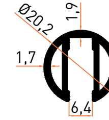
Profil No | 6122 Ağırlık / Weight: 0,350 kg/m
