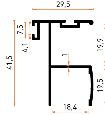
Profil No | 6996 Ağırlık / Weight: 0,364 kg/m
