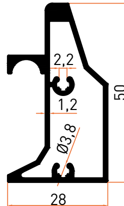
Profil No | 5971 Ağırlık / Weight: 0,659 kg/m
