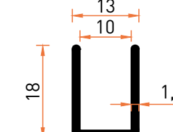
Profil No | 6330 Ağırlık / Weight: 0,184 kg/m
