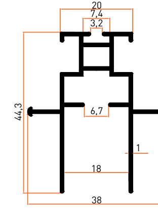
Profil No | 5640 Ağırlık / Weight: 0,442 kg/m
