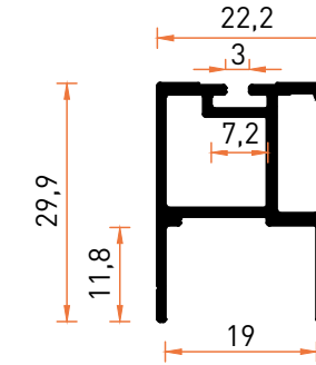
Profil No | 5367 Ağırlık / Weight: 0,454 kg/m
