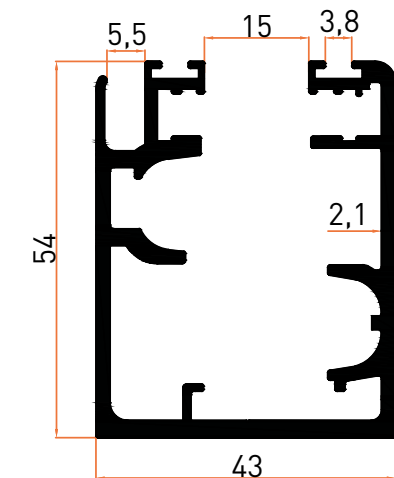
Profil No | 6145 Ağırlık / Weight: 1,358 kg/m
