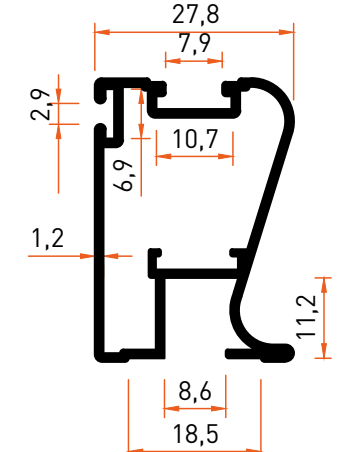
Profil No | 2225 Ağırlık / Weight: 0,565 kg/m
