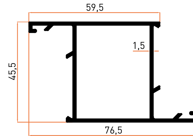
Profil No | 5529 Ağırlık / Weight: 0,935 kg/m
