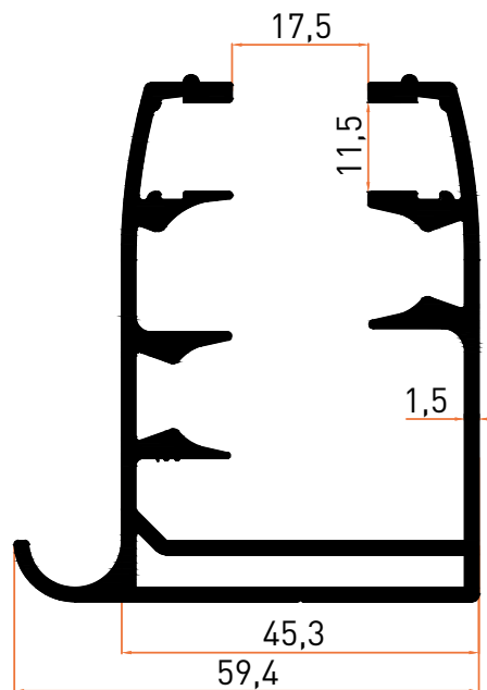
Profil No | 5893 Ağırlık / Weight: 1,578 kg/m
