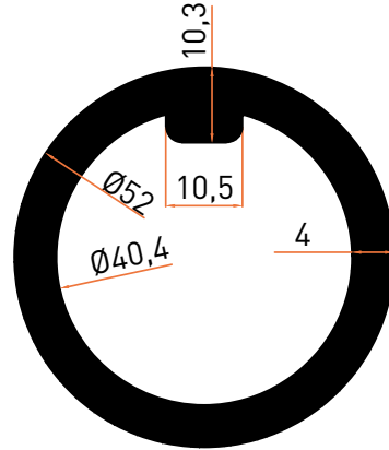
Profil No | 1610 Ağırlık / Weight: 1,628 kg/m
