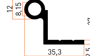
Profil No | 4050 Ağırlık / Weight: 0,461 kg/m
