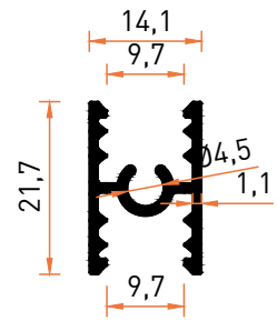
Profil No | 5203 Ağırlık / Weight: 0,244 kg/m
