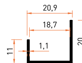
Profil No | 6240 Ağırlık / Weight: 0,150 kg/m
