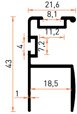
Profil No | 7159 Ağırlık / Weight: 0,395 kg/m
