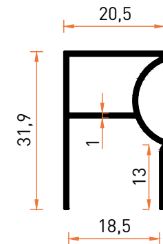
Profil No | 7420 Ağırlık / Weight: 0,276 kg/m
