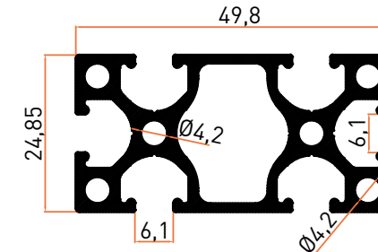
Profil No | 5209 Ağırlık / Weight: 1,032 kg/m
