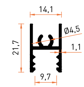
Profil No | 5206 Ağırlık / Weight: 0,234 kg/m
