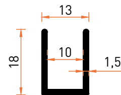
Profil No | 6330 Ağırlık / Weight: 0,184 kg/m
