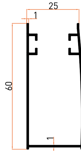
Profil No | 2586 Ağırlık / Weight: 0,441kg/m
