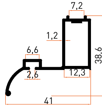
Profil No | 12114 Ağırlık / Weight: 0,409 kg/m
