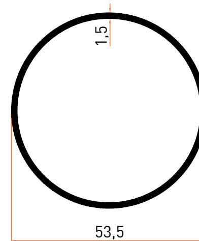
Profil No | 1618 Ağırlık / Weight: 0,664 kg/m
