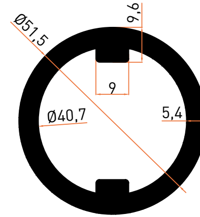
Profil No | 1635 Ağırlık / Weight: 2,314 kg/m
