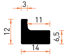
Profil No | 6248 Ağırlık / Weight: 0,293 kg/m
