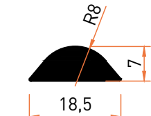
Profil No | 7231 Ağırlık / Weight: 0,242 kg/m
