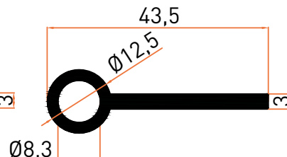
Profil No | 4003 Ağırlık / Weight: 0,455 kg/m
