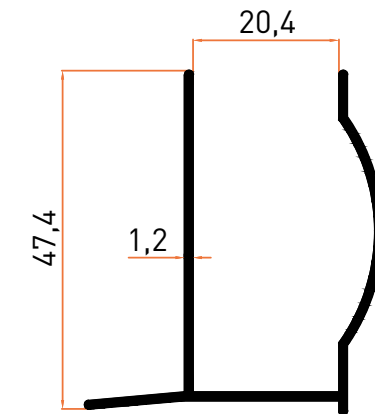
Profil No | 12226 Ağırlık / Weight: 0,423 kg/m
