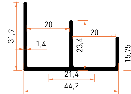
Profil No | 6901 Ağırlık / Weight: 0,422 kg/m
