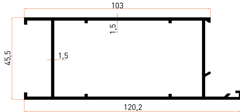
Profil No | 1010 Ağırlık / Weight: 1,334 kg/m
