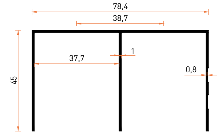
Profil No | 6776 Ağırlık / Weight: 0,563 kg/m
