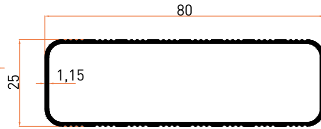
Profil No | 6721 Ağırlık / Weight: 0,555 kg/m
