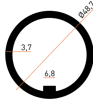
Profil No | 1642 Ağırlık / Weight: 1,477 kg/m
