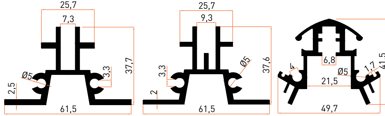
Profil No | 5262 Ağırlık / Weight: 1,038 kg/m
