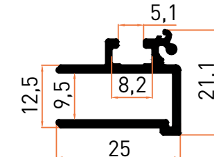
Profil No | 5671 Ağırlık / Weight: 0,327 kg/m
