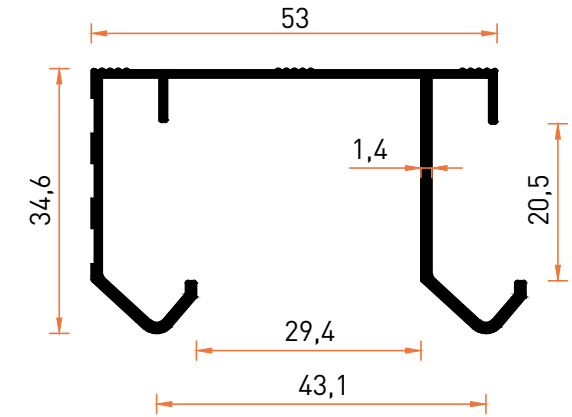
Profil No | 7704 Ağırlık / Weight: 0,506 kg/m
