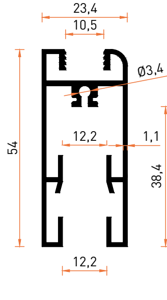
Profil No | 6752 Ağırlık / Weight: 0,670 kg/m
