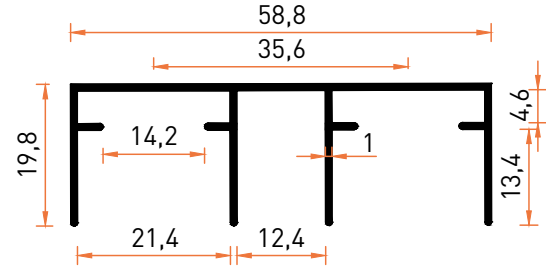
Profil No | 2561 Ağırlık / Weight: 0,373 kg/m
