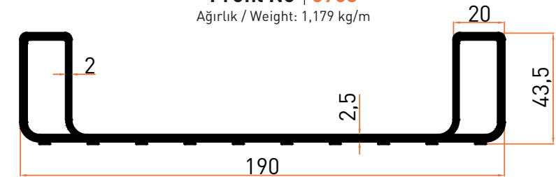
Profil No | 7024 Ağırlık / Weight: 2,548 kg/m
