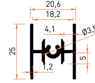
Profil No | 6808 Ağırlık / Weight: 0,319 kg/m
