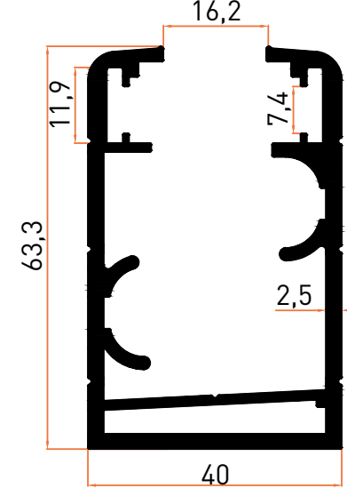
Profil No | 5358 Ağırlık / Weight: 1,627 kg/m
