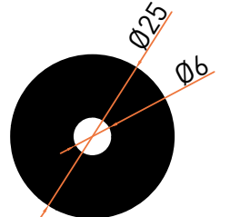
Profil No | 3001 Ağırlık / Weight: 1,254 kg/m
