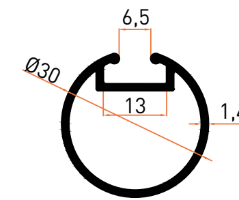
Profil No | 5841 Ağırlık / Weight: 0,403 kg/m
