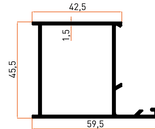
Profil No | 5527 Ağırlık / Weight: 0,813 kg/m
