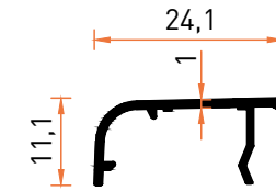
Profil No | 7381 Ağırlık / Weight: 0,130 kg/m
