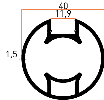
Profil No | 1641 Ağırlık / Weight: 0,752 kg/m
