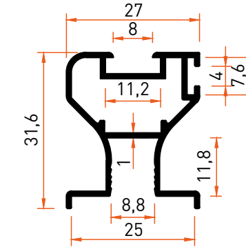
Profil No | 2221 Ağırlık / Weight: 0,378 kg/m
