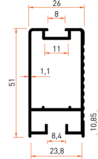
Profil No | 2234 Ağırlık / Weight: 0,597 kg/m
