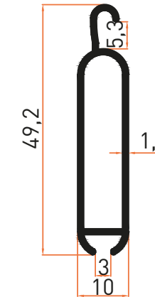
Profil No | 3101 Ağırlık / Weight: 0,347 kg/m
