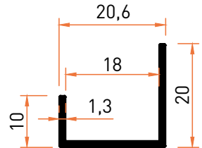
Profil No | 2567 Ağırlık / Weight: 0,174 kg/m
