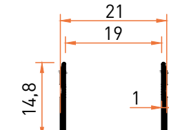
Profil No | 2624 Ağırlık / Weight: 0,125 kg/m
