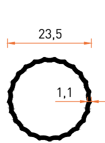
Profil No | 6431 Ağırlık / Weight: 0,195 kg/m
