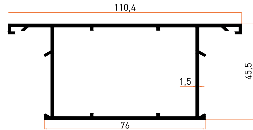
Profil No | 1009 Ağırlık / Weight: 1,203 kg/m
