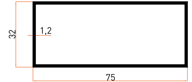
Profil No | 6029 Ağırlık / Weight: 0,680 kg/m
