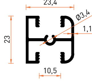
Profil No | 6740 Ağırlık / Weight: 0,346 kg/m
