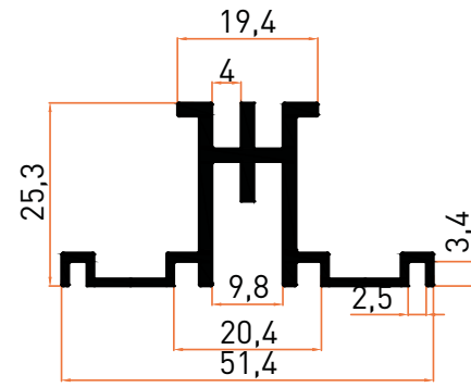
Profil No | 5686 Ağırlık / Weight: 0,550 kg/m
