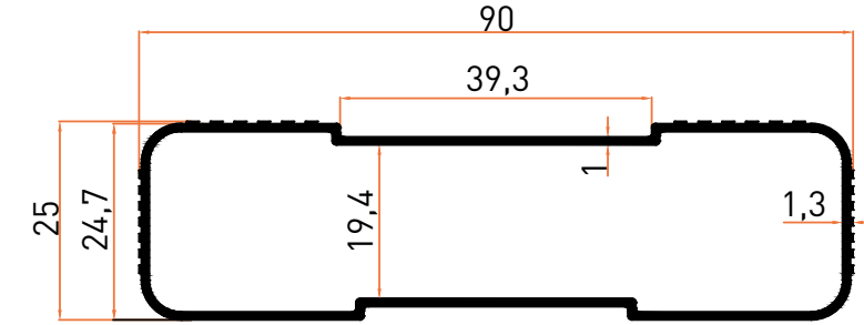
Profil No | 7113 Ağırlık / Weight: 0,631 kg/m
