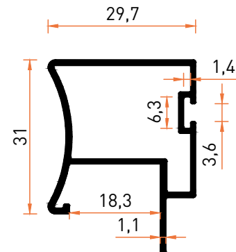
Profil No | 7305 Ağırlık / Weight: 0,416 kg/m
