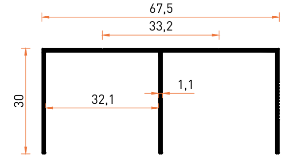
Profil No | 2209 Ağırlık / Weight: 0,456 kg/m
