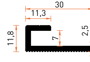
Profil No | 5427 Ağırlık / Weight: 0,298 kg/m
