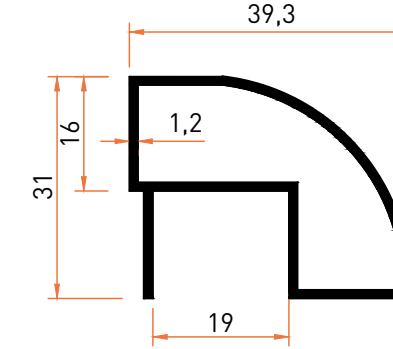
Profil No | 5367 Ağırlık / Weight: 0,454 kg/m
