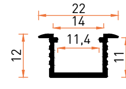
Profil No | 6138 Ağırlık / Weight: 0,133 kg/m
