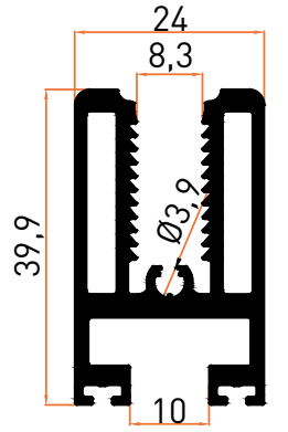
Profil No | 2248 Ağırlık / Weight: 0,948 kg/m
