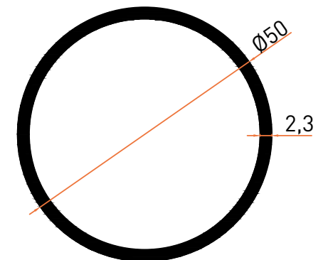
Profil No | 3013 Ağırlık / Weight: 0,934 kg/m
