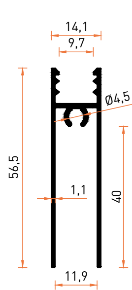
Profil No | 5207 Ağırlık / Weight: 0,442 kg/m
