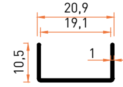
Profil No | 6514 Ağırlık / Weight: 0,096 kg/m
