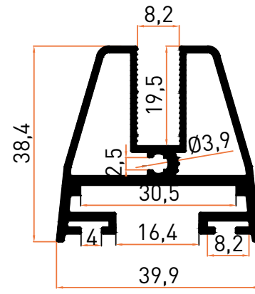
Profil No | 5894 Ağırlık / Weight: 0,873 kg/m
