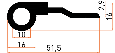
Profil No | 2581 Ağırlık / Weight: 0,744 kg/m
