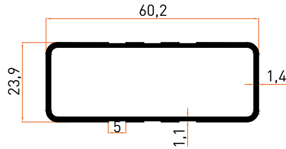
Profil No | 7098 Ağırlık / Weight: 0,576 kg/m
