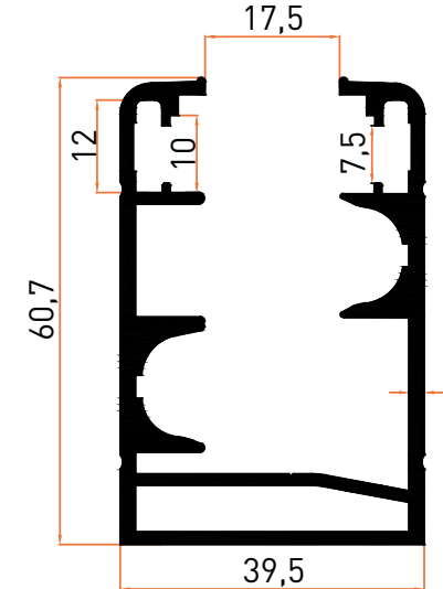
Profil No | 6688 Ağırlık / Weight: 1,382 kg/m
