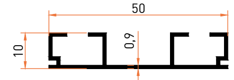
Profil No | 2849 Ağırlık / Weight: 0,261 kg/m
