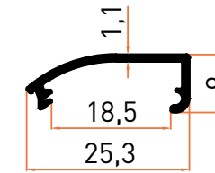
Profil No | 5672 Ağırlık / Weight: 0,120 kg/m
