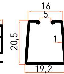
Profil No | 2769 Ağırlık / Weight: 0,186 kg/m
