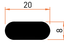
Profil No | 6956 Ağırlık / Weight: 0,369 kg/m
