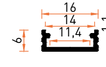
Profil No | 6139 Ağırlık / Weight: 0,081 kg/m
