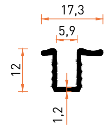
Profil No | 7405 Ağırlık / Weight: 0,118 kg/m
