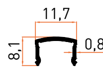
Profil No | 1608 Ağırlık / Weight: 0,062 kg/m
