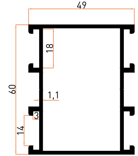
Profil No | 1401 Ağırlık / Weight: 0,875 kg/m
