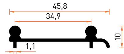
Profil No | 7419 Ağırlık / Weight: 0,295 kg/m
