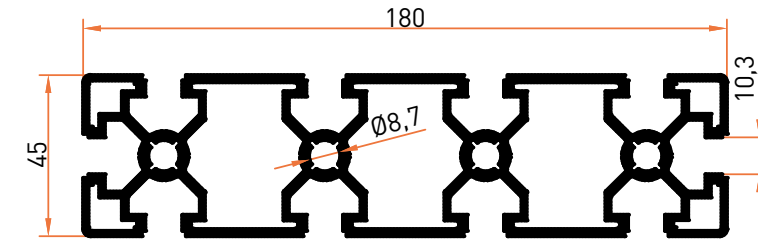
Profil No | 7198 Ağırlık / Weight: 4,543 kg/m
