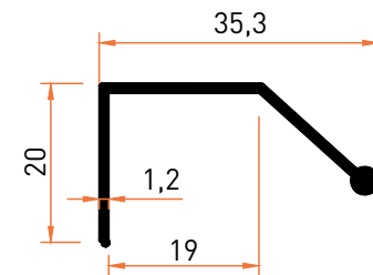
Profil No | 5289 Ağırlık / Weight: 0,205 kg/m
