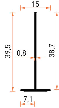
Profil No | 6735 Ağırlık / Weight: 0,113 kg/m
