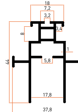
Profil No | 5195 Ağırlık / Weight: 0,456 kg/m
