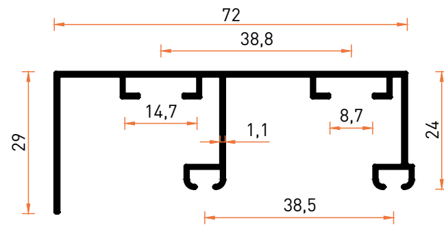
Profil No | 7571 Ağırlık / Weight: 0,552 kg/m
