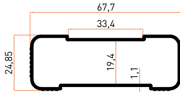
Profil No | 6147 Ağırlık / Weight: 0,542 kg/m
