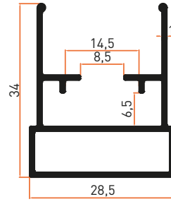
Profil No | 6212 Ağırlık / Weight: 0,385 kg/m
