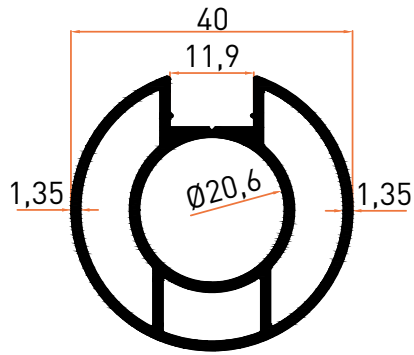
Profil No | 1609 Ağırlık / Weight: 0,803 kg/m
