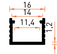
Profil No | 6140 Ağırlık / Weight: 0,122 kg/m
