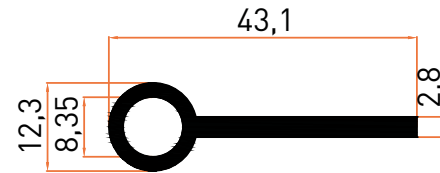
Profil No | 4024 Ağırlık / Weight: 0,408 kg/m
