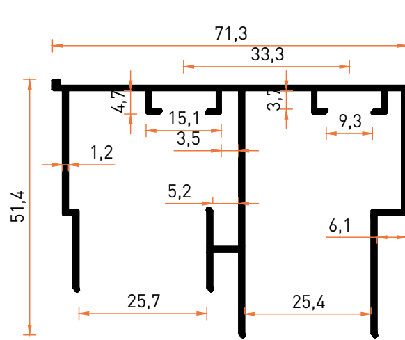
Profil No | 5551 Ağırlık / Weight: 0,832 kg/m
