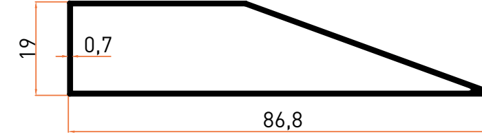
Profil No | 6461 Ağırlık / Weight: 0,369 kg/m
