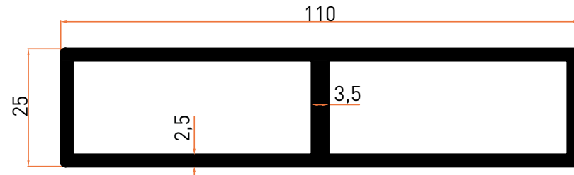
Profil No | 2615 Ağırlık / Weight: 2,014 kg/m
