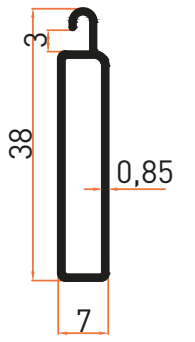
Profil No | 5241 Ağırlık / Weight: 0,190 kg/m
