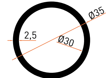
Profil No | 3007 Ağırlık / Weight: 0,692 kg/m
