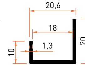
Profil No | 2567 Ağırlık / Weight: 0,174 kg/m
