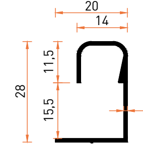
Profil No | 6806 Ağırlık / Weight: 0,198 kg/m
