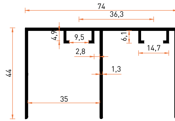
Profil No | 5457 Ağırlık / Weight: 0,798 kg/m
