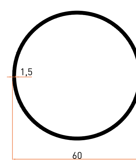
Profil No | 3004 Ağırlık / Weight: 0,747 kg/m
