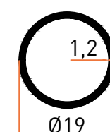
Profil No | 1606 Ağırlık / Weight: 0,182 kg/m
