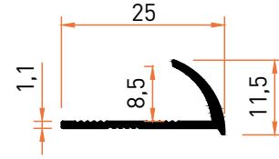
Profil No | 6916 Ağırlık / Weight: 0,111 kg/m
