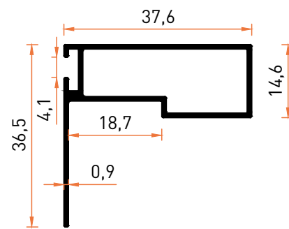
Profil No | 7108 Ağırlık / Weight: 0,327 kg/m
