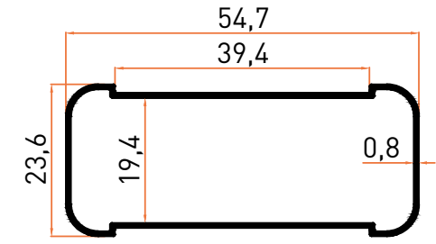
Profil No | 7110 Ağırlık / Weight: 0,327 kg/m
