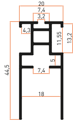
Profil No | 6214 Ağırlık / Weight: 0,388 kg/m
