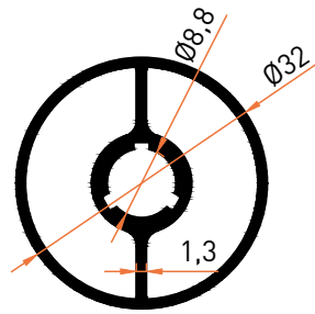
Profil No | 7143 Ağırlık / Weight: 0,549 kg/m
