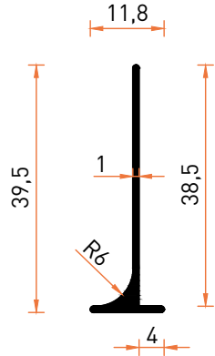
Profil No | 6733 Ağırlık / Weight: 0,156 kg/m
