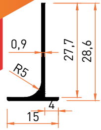
Profil No | 6723 Ağırlık / Weight: 0,119 kg/m
