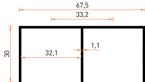
Profil No | 2209 Ağırlık / Weight: 0,456 kg/m
