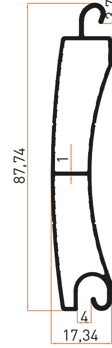
Profil No | 2755 Ağırlık / Weight: 0,621 kg/m
