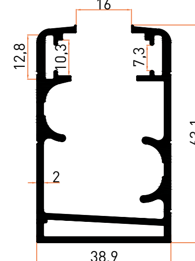
Profil No | 6684 Ağırlık / Weight: 1,372 kg/m
