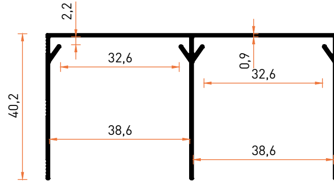
Profil No | 7585 Ağırlık / Weight: 0,531 kg/m
