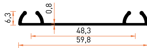
Profil No | 7415 Ağırlık / Weight: 0,184 kg/m
