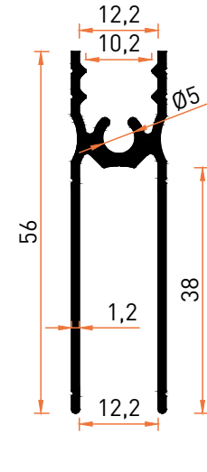
Profil No | 7019 Ağırlık / Weight: 0,487 kg/m
