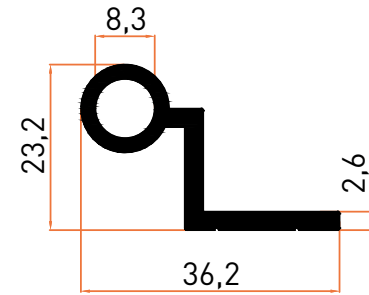
Profil No | 4023 Ağırlık / Weight: 0,445 kg/m
