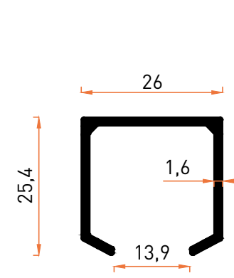
Profil No | 7040 Ağırlık / Weight: 0,346 kg/m
