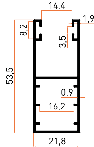
Profil No | 5061 Ağırlık / Weight: 0,430 kg/m
