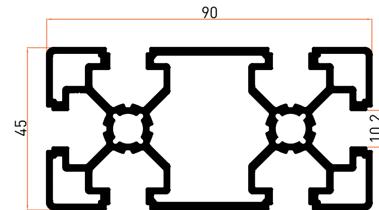
Profil No | 6993 Ağırlık / Weight: 2,434 kg/m
