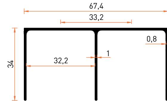
Profil No | 6612 Ağırlık / Weight: 0,453 kg/m
