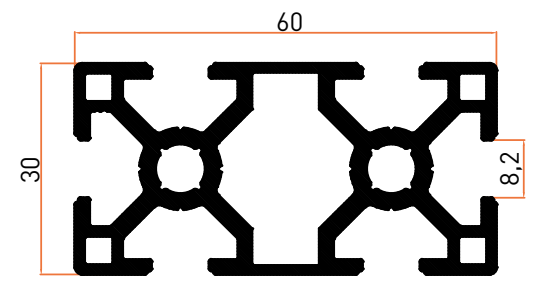
Profil No | 6988 Ağırlık / Weight: 1,488 kg/m
