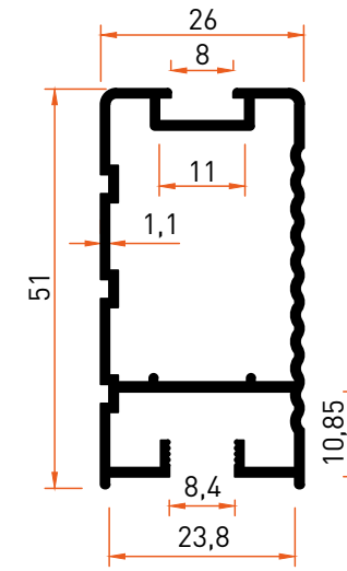
Profil No | 2235 Ağırlık / Weight: 0,592 kg/m
