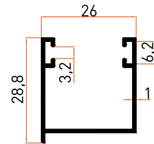
Profil No | 3102 Ağırlık / Weight: 0,266 kg/m
