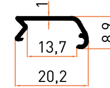
Profil No | 5764 Ağırlık / Weight: 0,097 kg/m
