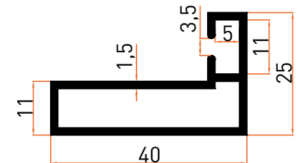
Profil No | 2242 Ağırlık / Weight: 0,508 kg/m
