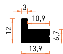
Profil No | 6077 Ağırlık / Weight: 0,295 kg/m
