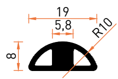
Profil No | 6717-2 Ağırlık / Weight: 0,222 kg/m
