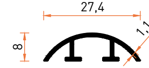
Profil No | 2658 Ağırlık / Weight: 0,155 kg/m
