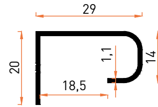
Profil No | 7057 Ağırlık / Weight: 0,194 kg/m
