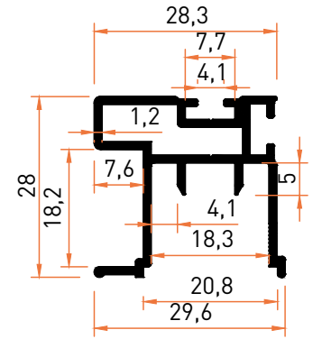
Profil No | 6809 Ağırlık / Weight: 0,445 kg/m
