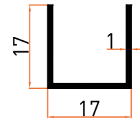
Profil No | 3103 Ağırlık / Weight: 0,133 kg/m
