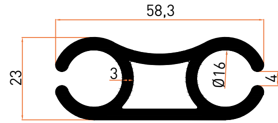
Profil No | 6954 Ağırlık / Weight: 1,400 kg/m
