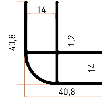
Profil No | 12440 Ağırlık / Weight: 0,493 kg/m
