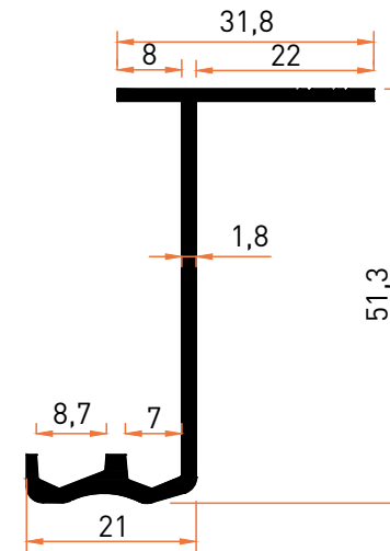
Profil No | 6900 Ağırlık / Weight: 0,503 kg/m
