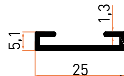
Profil No | 1021 Ağırlık / Weight: 0,145 kg/m
