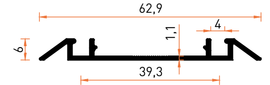
Profil No | 7583 Ağırlık / Weight: 0,264 kg/m
