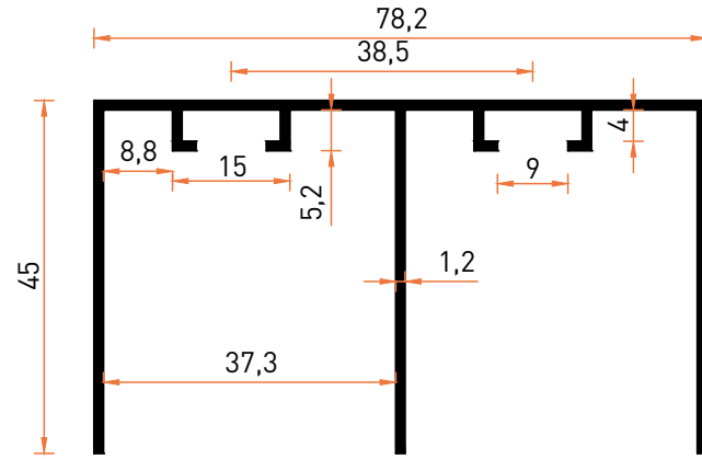
Profil No | 6736 Ağırlık / Weight: 0,772 kg/m
