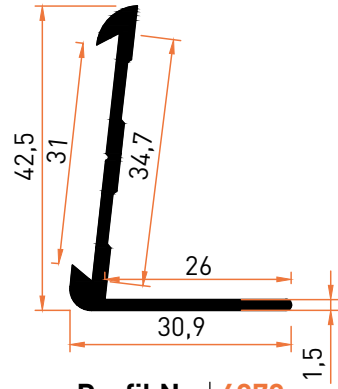
Profil No | 6878 Ağırlık / Weight: 0,372 kg/m
