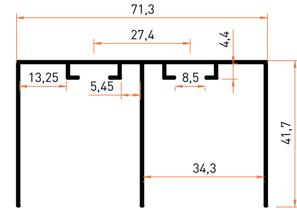
Profil No | 7228 Ağırlık / Weight: 0,540 kg/m
