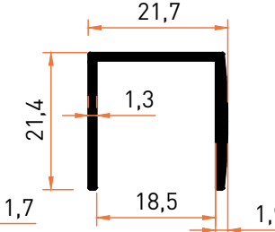
Profil No | 5329 Ağırlık / Weight: 0,239 kg/m
