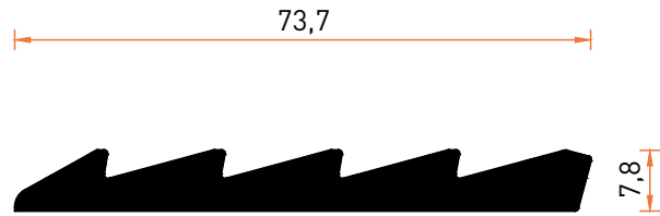
Profil No | 5049 Ağırlık / Weight: 1,183 kg/m
