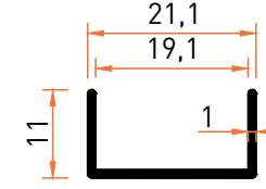
Profil No | 5932 Ağırlık / Weight: 0,111 kg/m
