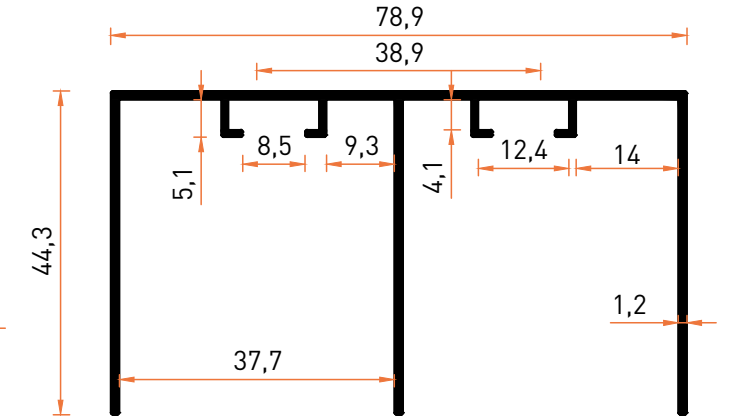
Profil No | 7022 Ağırlık / Weight: 0,752 kg/m
