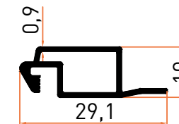
Profil No | 2512 Ağırlık / Weight: 0,186 kg/m
