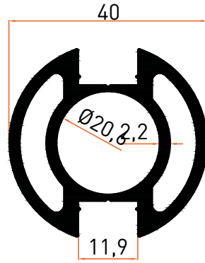
Profil No | 1603 Ağırlık / Weight: 1,188 kg/m
