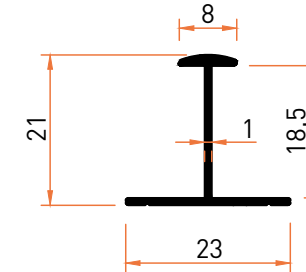
Profil No | 6768 Ağırlık / Weight: 0,138 kg/m
