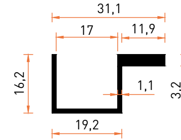
Profil No | 5474 Ağırlık / Weight: 0,250 kg/m
