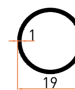
Profil No | 3006 Ağırlık / Weight: 0,153 kg/m
