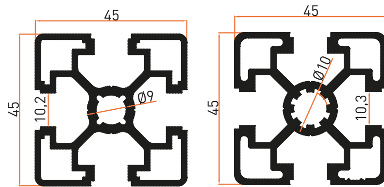
Profil No | 6818 Ağırlık / Weight: 1,480 kg/m
