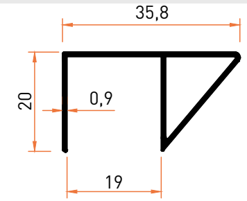
Profil No | 6814 Ağırlık / Weight: 0,236 kg/m
