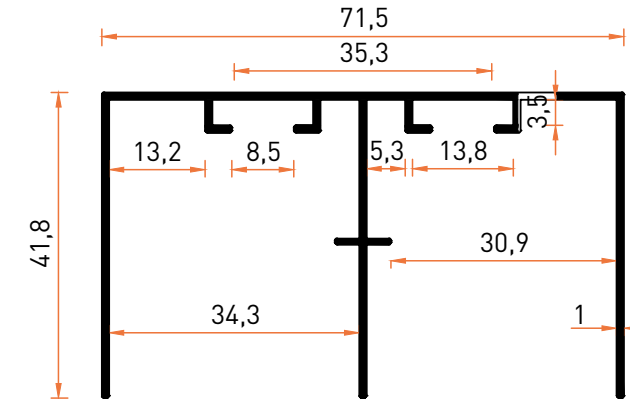
Profil No | 7023 Ağırlık / Weight: 0,616 kg/m
