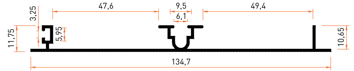
Profil No | 7077 Ağırlık / Weight: 0,574 kg/m
