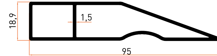
Profil No | 7119 Ağırlık / Weight: 0,849 kg/m
