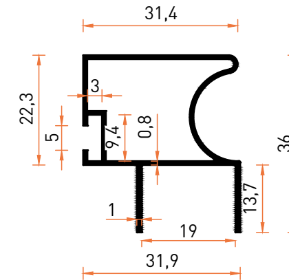
Profil No | 7576 Ağırlık / Weight: 0,328 kg/m
