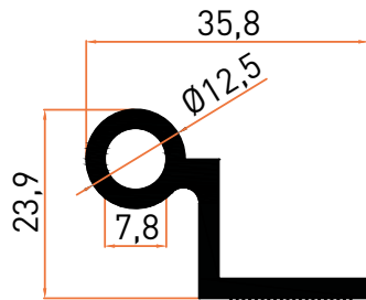
Profil No | 4010 Ağırlık / Weight: 0,475 kg/m
