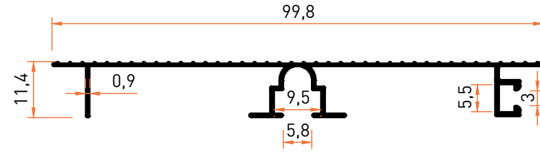
Profil No | 7169 Ağırlık / Weight: 0,381 kg/m
