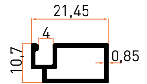
Profil No | 2504 Ağırlık / Weight: 0,152 kg/m
