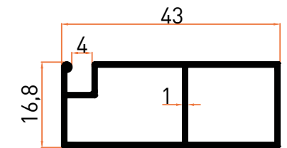
Profil No | 2505 Ağırlık / Weight: 0,373 kg/m
