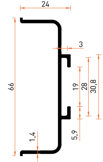
Profil No | 6166 Ağırlık / Weight: 0,442 kg/m
