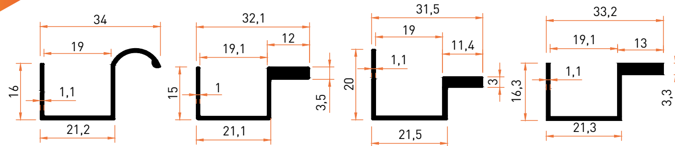
Profil No | 2204 Ağırlık / Weight: 0,204 kg/m Profil No | 5931 Ağırlık / Weight: 0,236 kg/m Profil No | 6541 Ağırlık / Weight: 0,241 kg/m Profil No | 5472 Ağırlık / Weight: 0,260 kg/m
