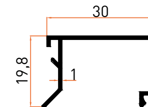
Profil No | 1006 Ağırlık / Weight: 0,205 kg/m
