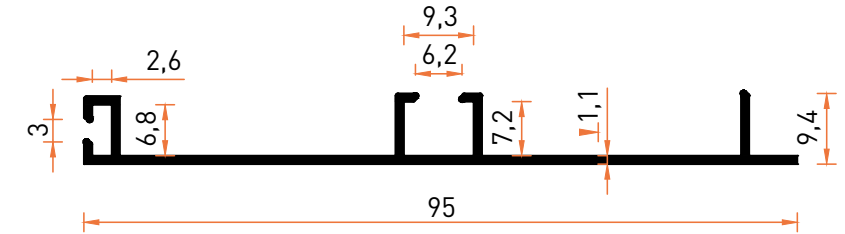
Profil No | 6774 Ağırlık / Weight: 0,411 kg/m
