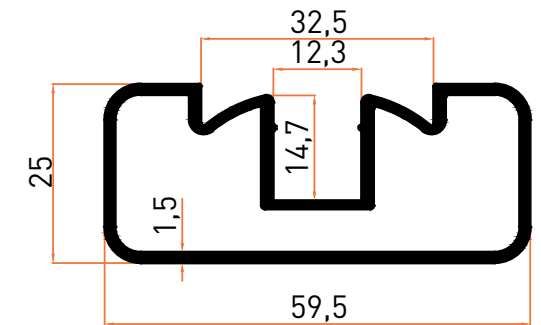
Profil No | 6291 Ağırlık / Weight: 0,799 kg/m
