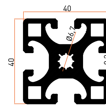
Profil No | 6985 Ağırlık / Weight: 1,875 kg/m
