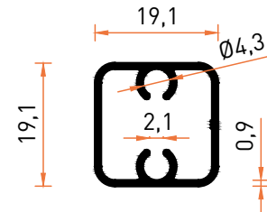
Profil No | 7771 Ağırlık / Weight: 0,224 kg/m
