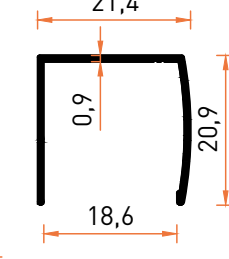
Profil No | 7412 Ağırlık / Weight: 0,158 kg/m
