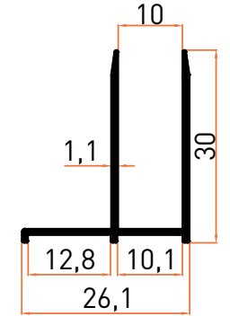
Profil No | 6918 Ağırlık / Weight: 0,240 kg/m
