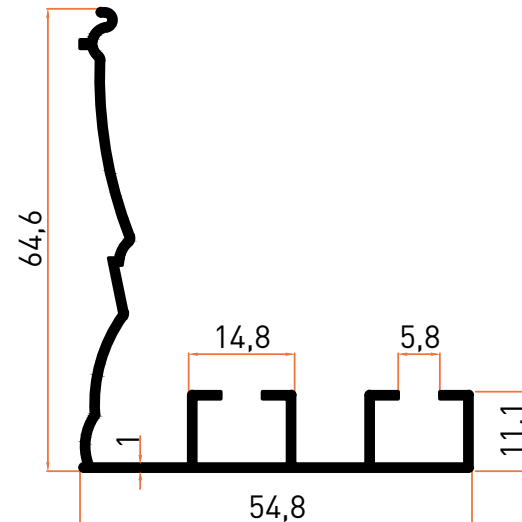
Profil No | 2545 Ağırlık / Weight: 0,503 kg/m
