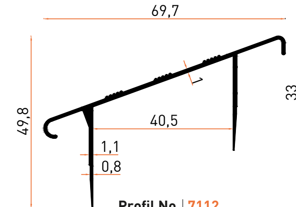
Profil No | 7112 Ağırlık / Weight: 0,390 kg/m
