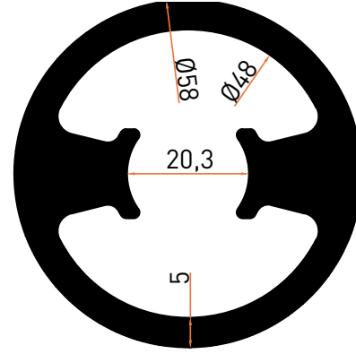
Profil No | 1632 Ağırlık / Weight: 3,133 kg/m
