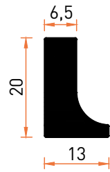
Profil No | 7021 Ağırlık / Weight: 0,420 kg/m
