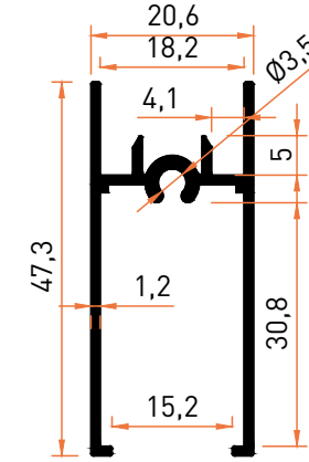
Profil No | 6807 Ağırlık / Weight: 0,448 kg/m
