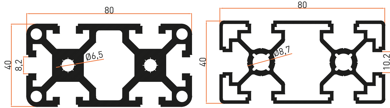
Profil No | 7200 Ağırlık / Weight: 3,252 kg/m
