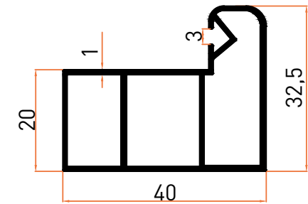
Profil No | 2247 Ağırlık / Weight: 0,509 kg/m
