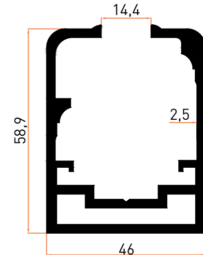
Profil No | 2250 Ağırlık / Weight: 1,817 kg/m
