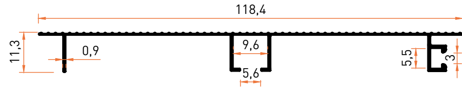
Profil No | 7168 Ağırlık / Weight: 0,368 kg/m
