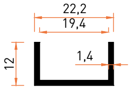
Profil No | 2223 Ağırlık / Weight: 0,165 kg/m
