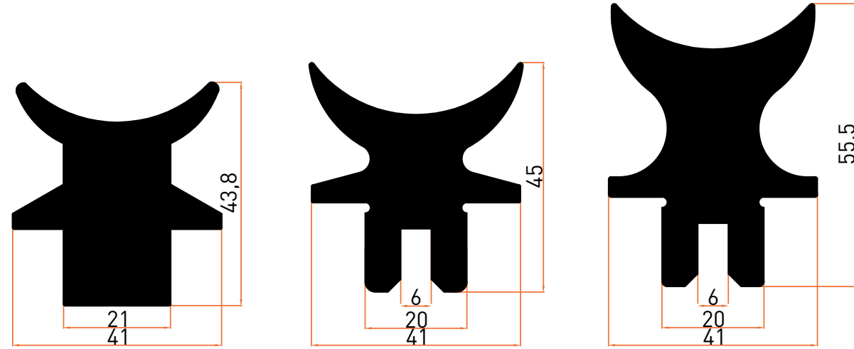
Profil No | 5236 Ağırlık / Weight: 2,685 kg/m
