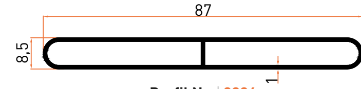
Profil No | 2926 Ağırlık / Weight: 0,507 kg/m
