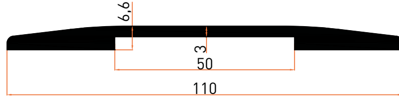
Profil No | 2571 Ağırlık / Weight: 1,267 kg/m
