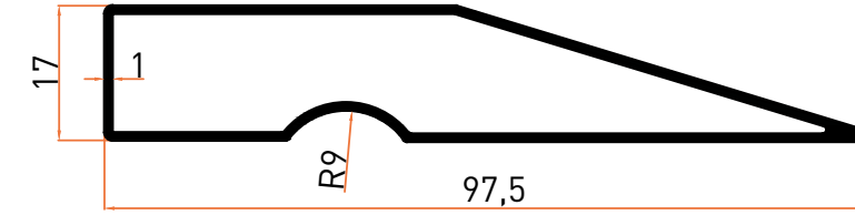
Profil No | 5238 Ağırlık / Weight: 0,578 kg/m
