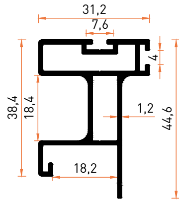
Profil No | 7008 Ağırlık / Weight: 0,596 kg/m
