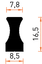
Profil No | 6256 Ağırlık / Weight: 0,282 kg/m
