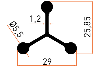
Profil No | 6263 Ağırlık / Weight: 0,304 kg/m
