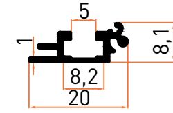
Profil No | 5765 Ağırlık / Weight: 0,124 kg/m
