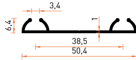
Profil No | 6741 Ağırlık / Weight: 0,210 kg/m
