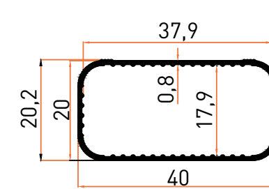
Profil No | 7109 Ağırlık / Weight: 0,257 kg/m
