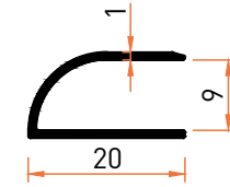
Profil No | 6877 Ağırlık / Weight: 0,120 kg/m
