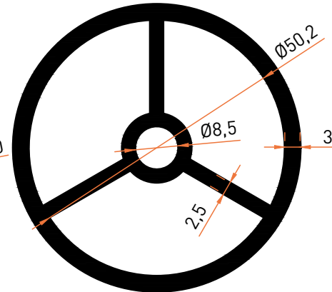
Profil No | 6690 Ağırlık / Weight: 1,965 kg/m
