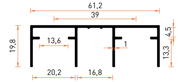
Profil No | 6795 Ağırlık / Weight: 0,407 kg/m
