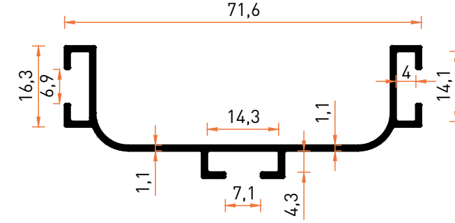
Profil No | 7675 Ağırlık / Weight: 0,448 kg/m
