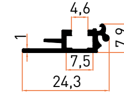
Profil No | 6725 Ağırlık / Weight: 0,138 kg/m
