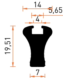
Profil No | 5523 Ağırlık / Weight: 0,399 kg/m
