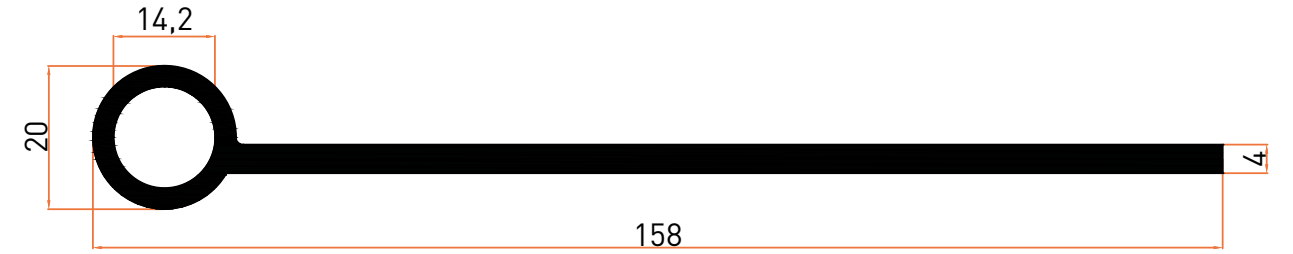
Profil No | 4016 Ağırlık / Weight: 1,925 kg/m
