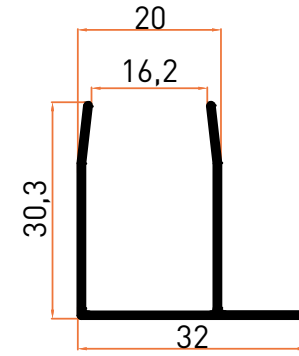
Profil No | 5784 Ağırlık / Weight: 0,244 kg/m
