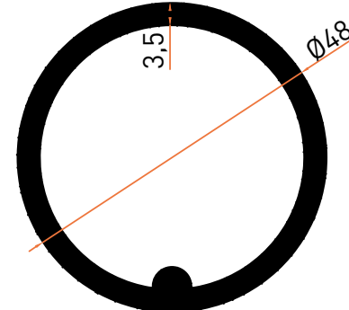
Profil No | 5669 Ağırlık / Weight: 1,372 kg/m
