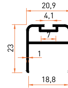
Profil No | 5300 Ağırlık / Weight: 0,241 kg/m
