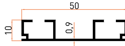
Profil No | 2849 Ağırlık / Weight: 0,260 kg/m
