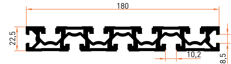
Profil No | 7199 Ağırlık / Weight: 4,065 kg/m
