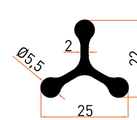
Profil No | 6296 Ağırlık / Weight: 0,347 kg/m
