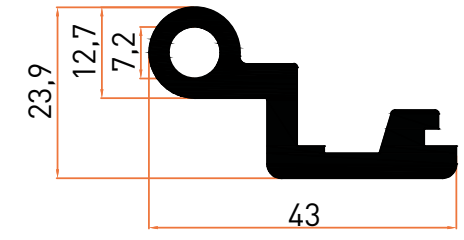
Profil No | 4052 Ağırlık / Weight: 0,819 kg/m
