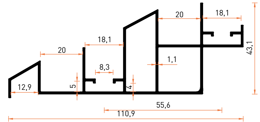
Profil No | 2836 Ağırlık / Weight: 1,005 kg/m
