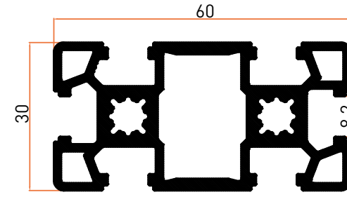
Profil No | 6978 Ağırlık / Weight: 1,545 kg/m
