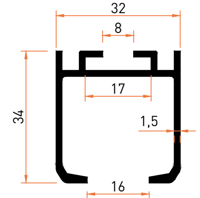
Profil No | 7237 Ağırlık / Weight: 0,533 kg/m
