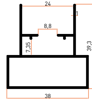
Profil No | 5639 Ağırlık / Weight: 0,455 kg/m
