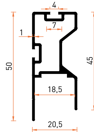
Profil No | 7162 Ağırlık / Weight: 0,436 kg/m
