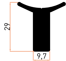
Profil No | 6134 Ağırlık / Weight: 0,784 kg/m
