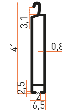
Profil No | 5060 Ağırlık / Weight: 0,202 kg/m
