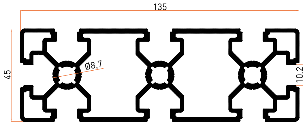
Profil No | 6981 Ağırlık / Weight: 3,501 kg/m
