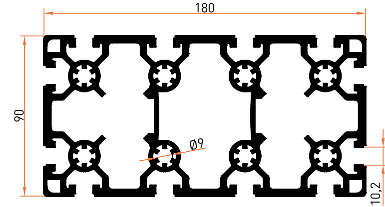
Profil No | 7197 Ağırlık / Weight: 9,484 kg/m
