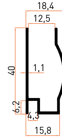
Profil No | 6668 Ağırlık / Weight: 0,299 kg/m
