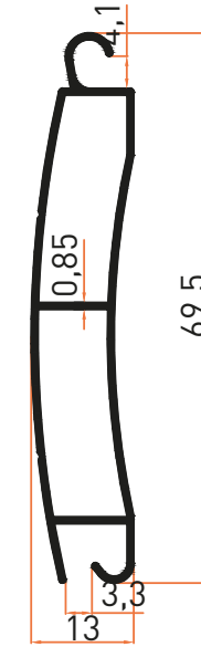
Profil No | 5763 Ağırlık / Weight: 0,387 kg/m
