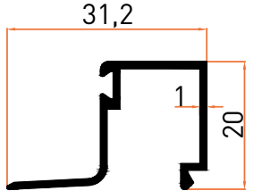
Profil No | 1007 Ağırlık / Weight: 0,211 kg/m
