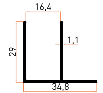
Profil No | 6277 Ağırlık / Weight: 0,269 kg/m
