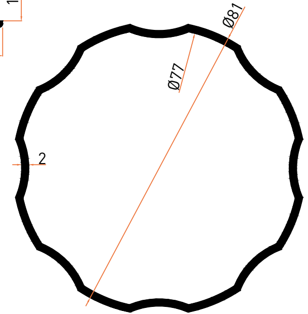
Profil No | 5404 Ağırlık / Weight: 1,359 kg/m
