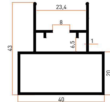
Profil No | 5196 Ağırlık / Weight: 0,495 kg/m
