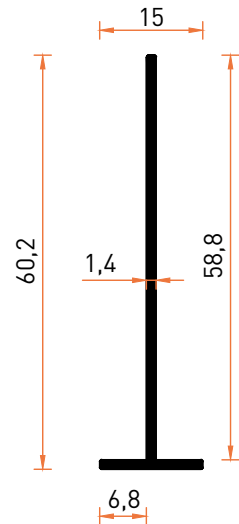
Profil No | 6616 Ağırlık / Weight: 0,279 kg/m
