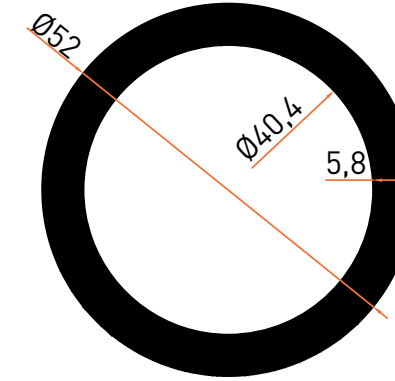
Profil No | 1617 Ağırlık / Weight: 2,281 kg/m
