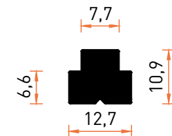
Profil No | 7531 Ağırlık / Weight: 0,314 kg/m
