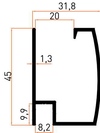
Profil No | 5970 Ağırlık / Weight: 0,474 kg/m
