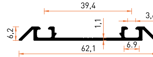
Profil No | 7185 Ağırlık / Weight: 0,287 kg/m
