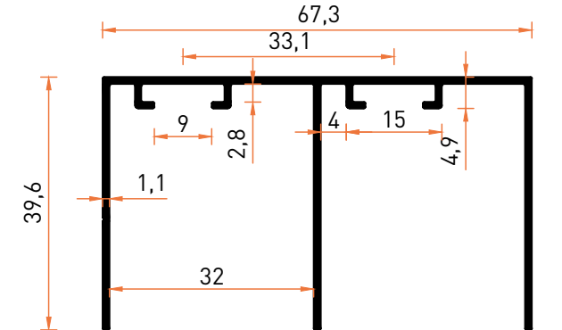
Profil No | 6550 Ağırlık / Weight: 0,607 kg/m
