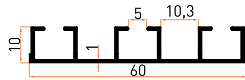
Profil No | 5786 Ağırlık / Weight: 0,358 kg/m
