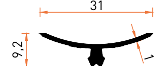
Profil No | 6714 Ağırlık / Weight: 0,130 kg/m
