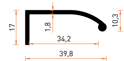
Profil No | 7677 Ağırlık / Weight: 0,289 kg/m
