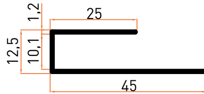
Profil No | 2674 Ağırlık / Weight: 0,260 kg/m
