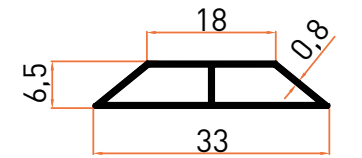
Profil No | 6459 Ağırlık / Weight: 0,146 kg/m
