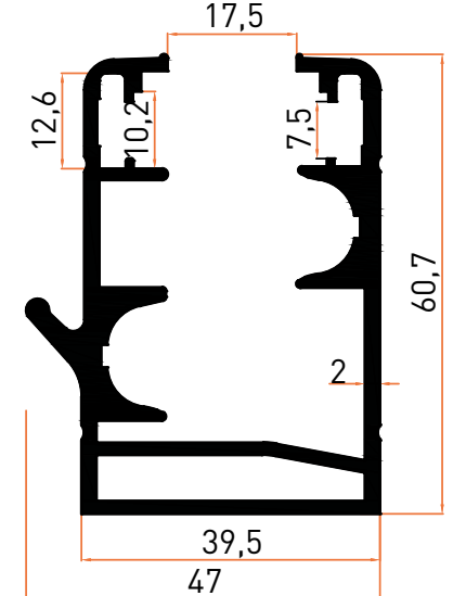
Profil No | 6687 Ağırlık / Weight: 1,462 kg/m
