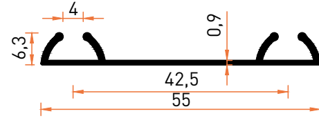
Profil No | 2589 Ağırlık / Weight: 0,217 kg/m
