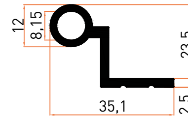
Profil No | 4049 Ağırlık / Weight: 0,434 kg/m
