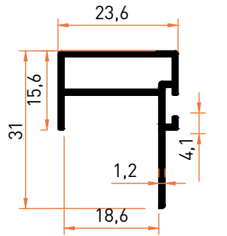
Profil No | 5040 Ağırlık / Weight: 0,307 kg/m
