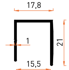
Profil No | 7058 Ağırlık / Weight: 0,161 kg/m
