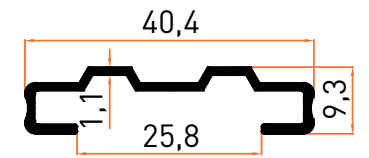
Profil No | 6031 Ağırlık / Weight: 0,211 kg/m
