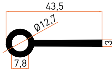
Profil No | 4012 Ağırlık / Weight: 0,458 kg/m
