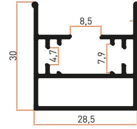
Profil No | 6213 Ağırlık / Weight: 0,396 kg/m
