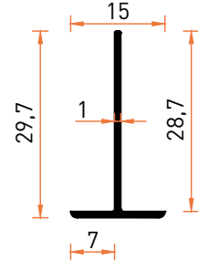
Profil No | 6724 Ağırlık / Weight: 0,117 kg/m
