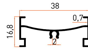
Profil No | 5610 Ağırlık / Weight: 0,187 kg/m
