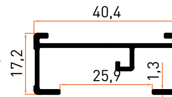
Profil No | 6030 Ağırlık / Weight: 0,317 kg/m
