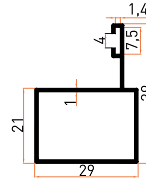
Profil No | 2243 Ağırlık / Weight: 0,330 kg/m
