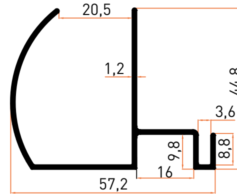
Profil No | 5979 Ağırlık / Weight: 0,525 kg/m
