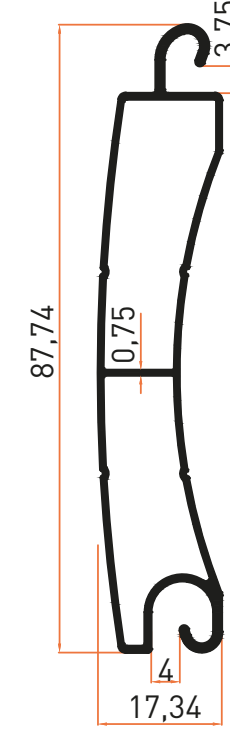
Profil No | 5644 Ağırlık / Weight: 0,512 kg/m
