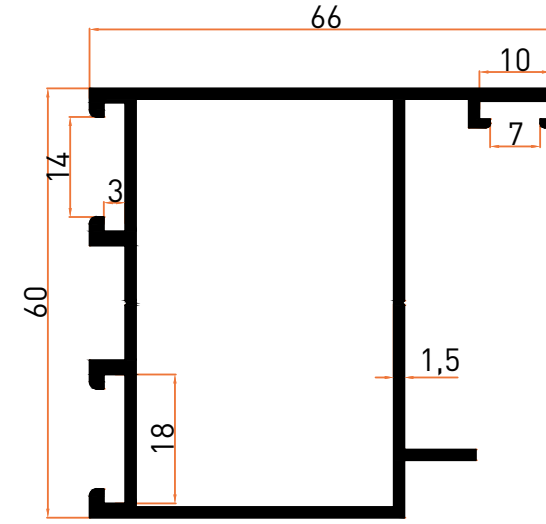
Profil No | 1400 Ağırlık / Weight: 1,109 kg/m
