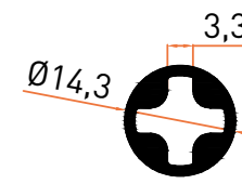
Profil No | 5607 Ağırlık / Weight: 0,247 kg/m
