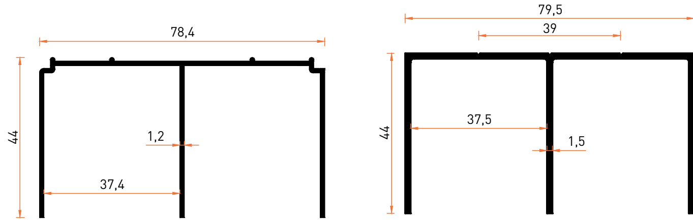
Profil No | 7009 Ağırlık / Weight: 0,672 kg/m
