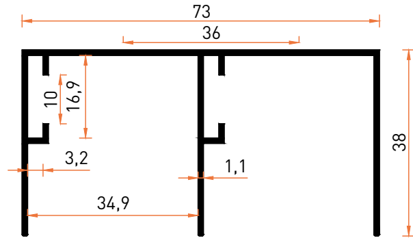
Profil No | 5039 Ağırlık / Weight: 0,614 kg/m
