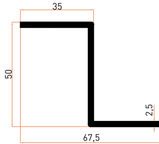
Profil No | 2614 Ağırlık / Weight: 0,804 kg/m
