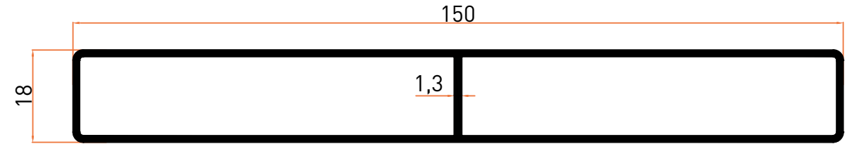
Profil No | 6789 Ağırlık / Weight: 1,211 kg/m
