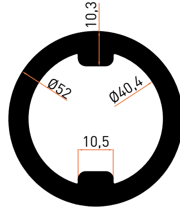
Profil No | 1612 Ağırlık / Weight: 2,514 kg/m
