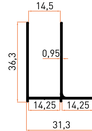
Profil No | 11668 Ağırlık / Weight: 0,271 kg/m
