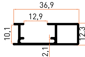
Profil No | 12115 Ağırlık / Weight: 0,279 kg/m
