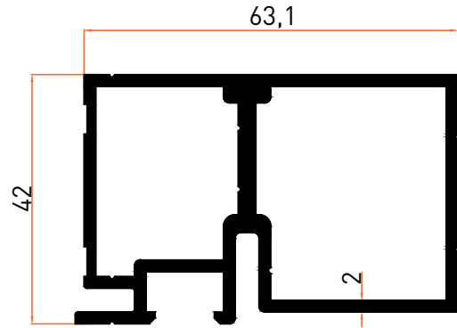
Profil No | 2620 Ağırlık / Weight: 1,537 kg/m
