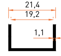
Profil No | 5473 Ağırlık / Weight: 0,128 kg/m
