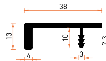
Profil No | 7081 Ağırlık / Weight: 0,395 kg/m
