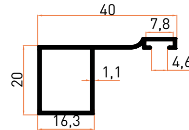
Profil No | 2507 Ağırlık / Weight: 0,295 kg/m
