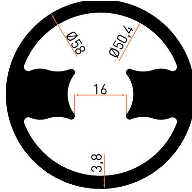
Profil No | 1619 Ağırlık / Weight: 2,691 kg/m
