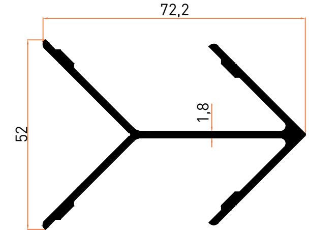
Profil No | 1012 Ağırlık / Weight: 0,973 kg/m
