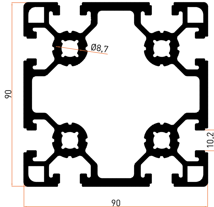
Profil No | 6987 Ağırlık / Weight: 5,640 kg/m
