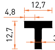
Profil No | 5777 Ağırlık / Weight: 0,185 kg/m
