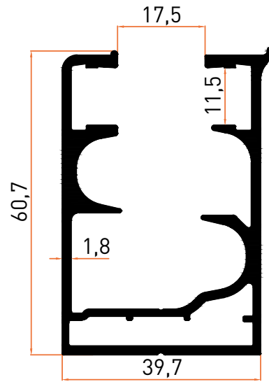
Profil No | 5888 Ağırlık / Weight: 1,334 kg/m
