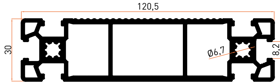
Profil No | 6982 Ağırlık / Weight: 2,482 kg/m
