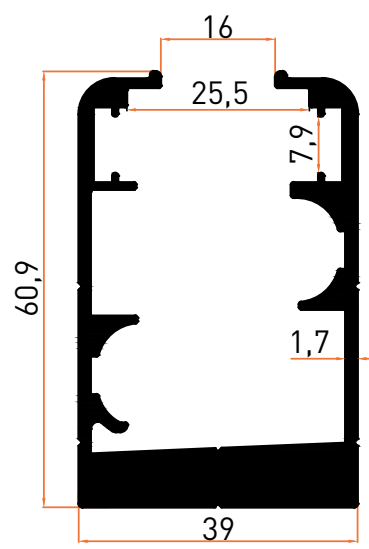
Profil No | 5058 Ağırlık / Weight: 1,232 kg/m
