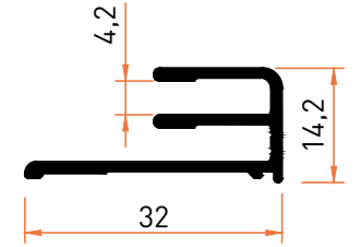
Profil No | 7178 Ağırlık / Weight: 0,265 kg/m
